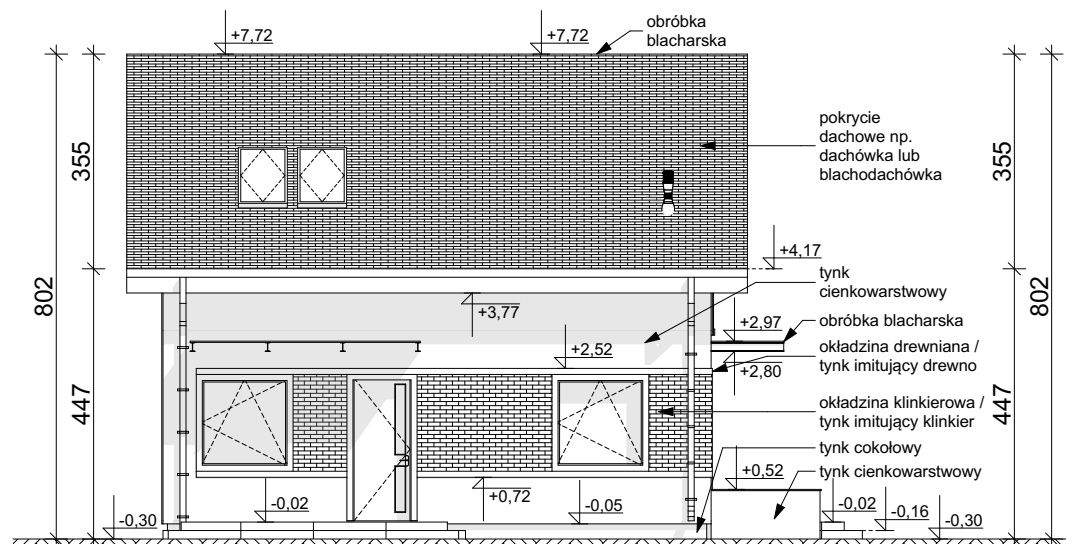
ELEWACJA FRONTOWA
