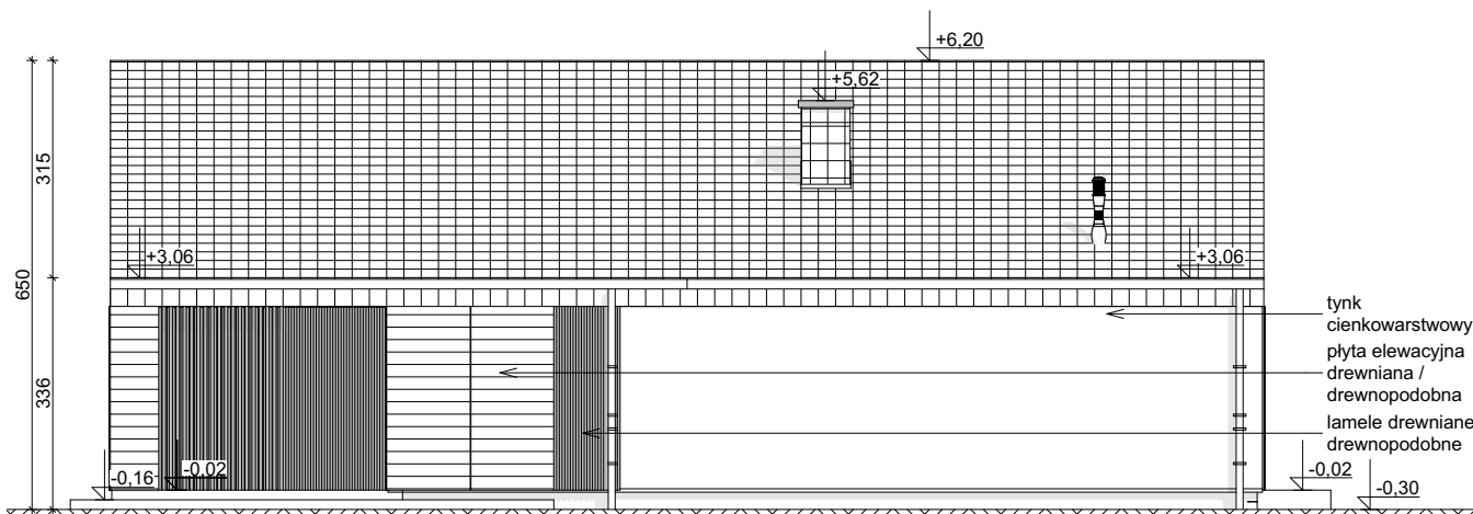
ELEVACJA BOCZNA
