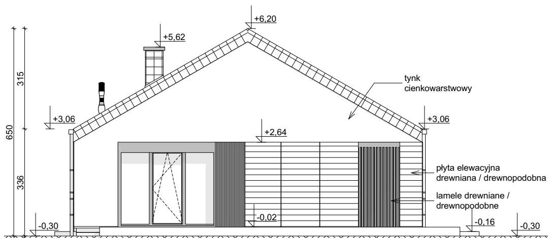
ELEVACJA OGRODOWA
