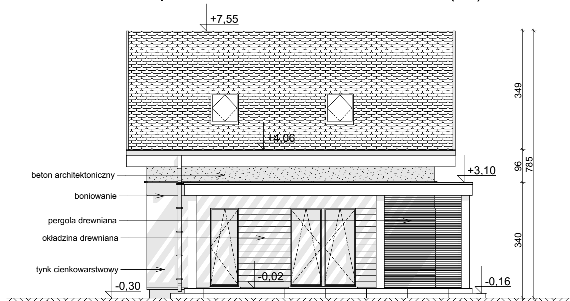
ELEWACJA OGRODOWA
