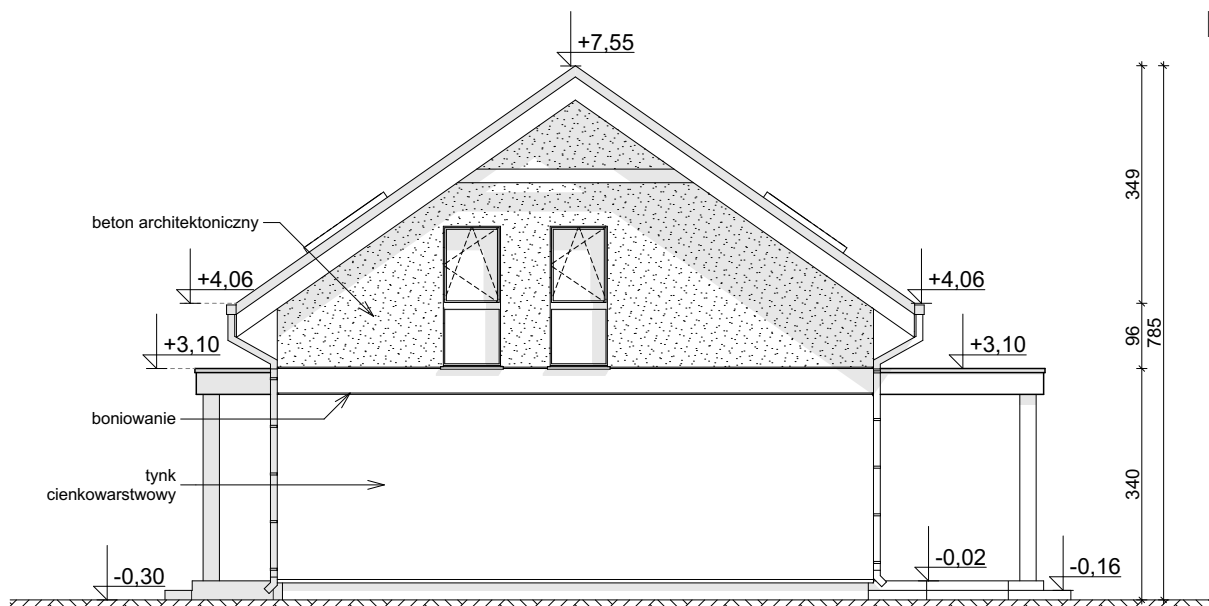
ELEWACJA BOCZNA
