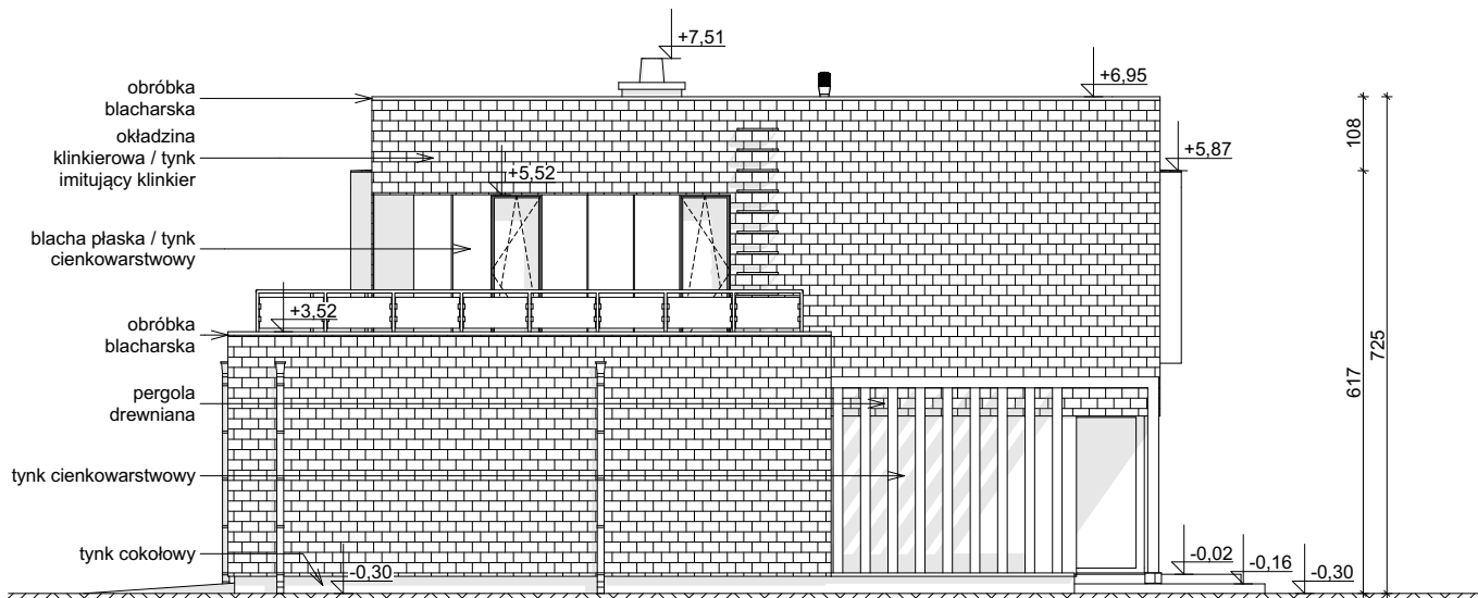
ELEWACJA BOCZNA
