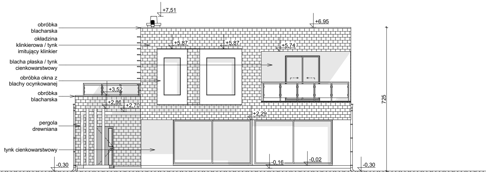
ELEWACJA OGRODOWA
