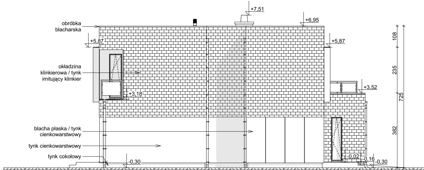
ELEWACJA BOCZNA
