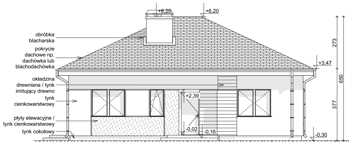
ELEWACJA FRONTOWA
