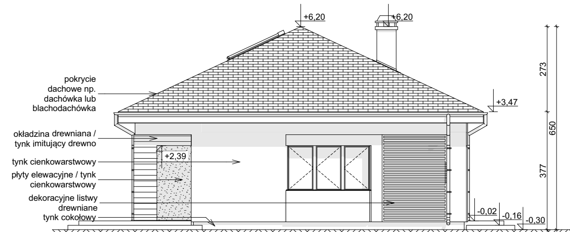
ELEWACJA BOCZNA
