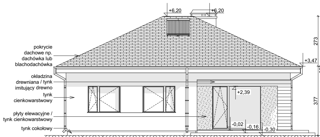
ELEWACJA OGRODOWA
