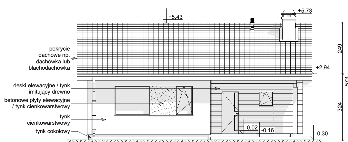
ELEWACJA FRONTOWA
