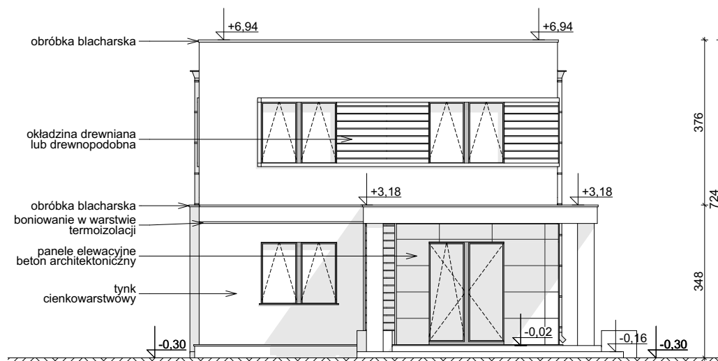
ELEVACJA OGRODOWA
