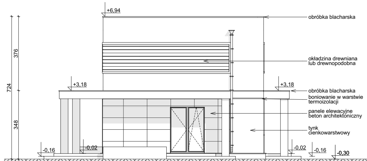
ELEWACJA BOCZNA
