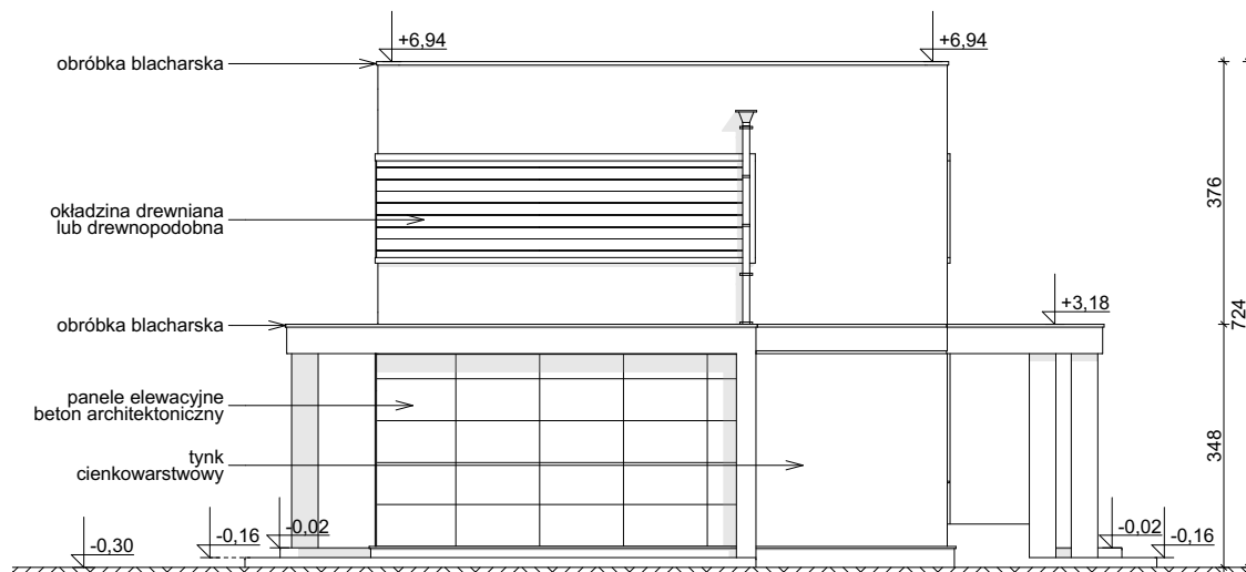
ELEVACJA BOCZNA
