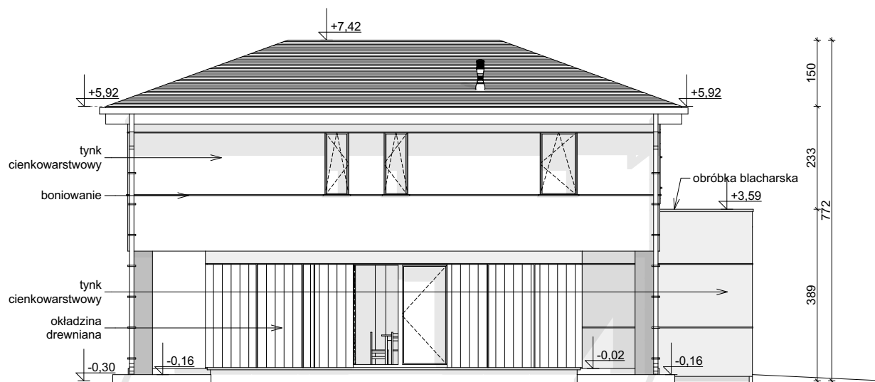
ELEWACJA BOCZNA
