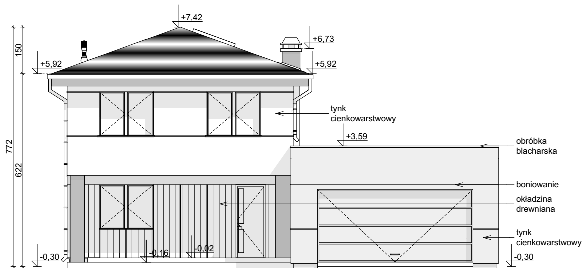
ELEWACJA FRONTOWA
