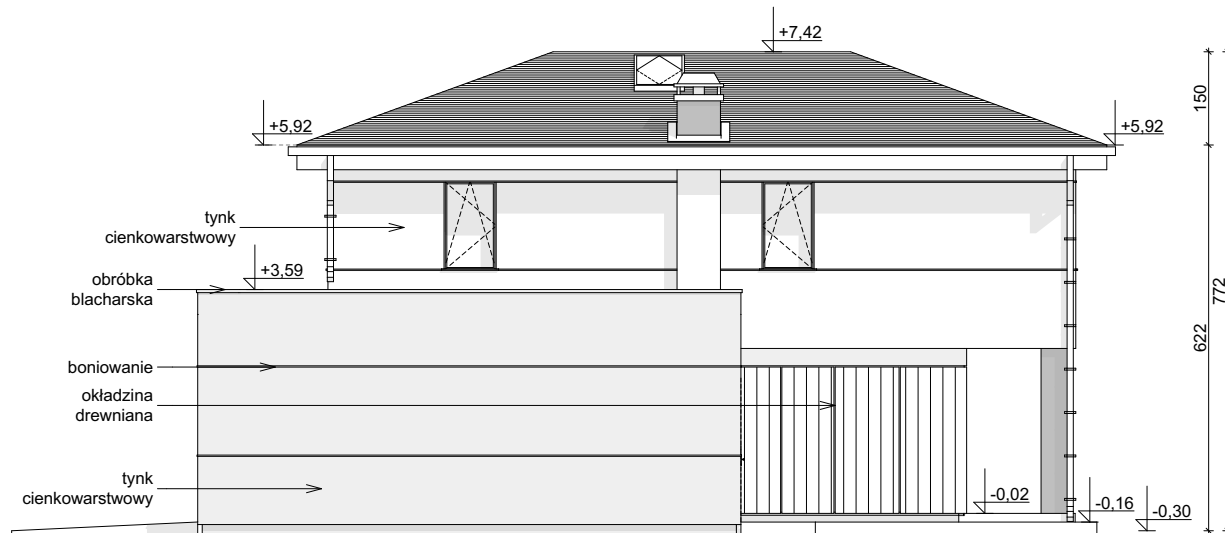
ELEWACJA BOCZNA
