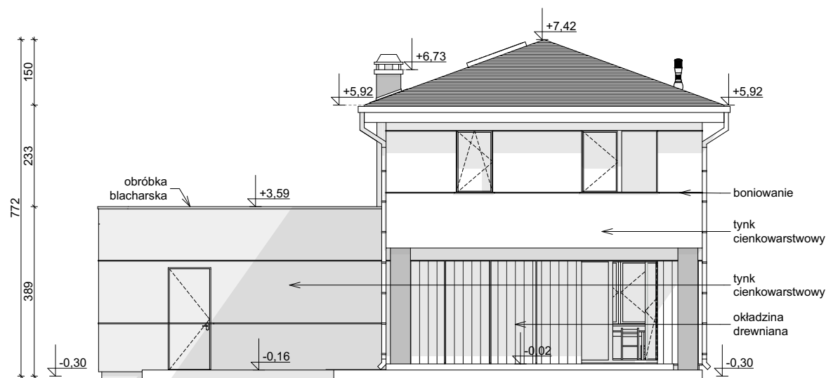
ELEWACJA OGRODOWA
