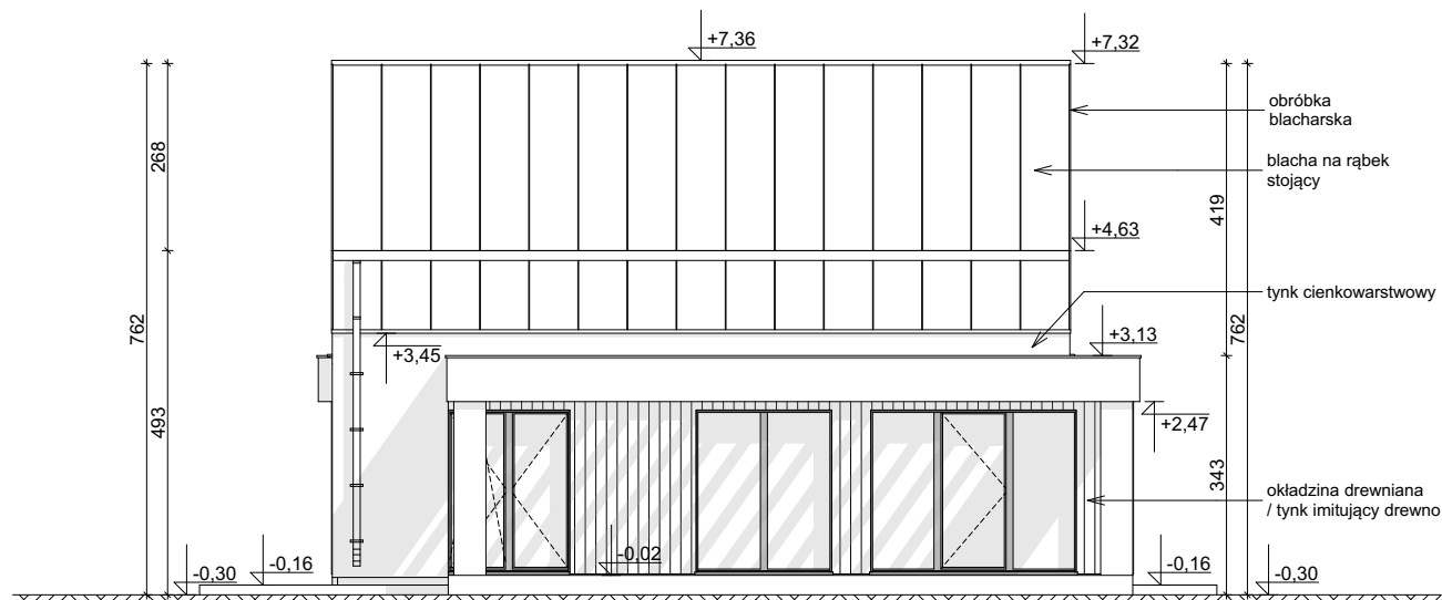
ELEWACJA OGRODOWA
