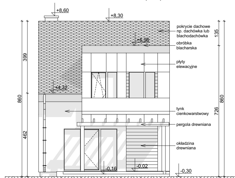
ELEWACJA OGRODOWA
