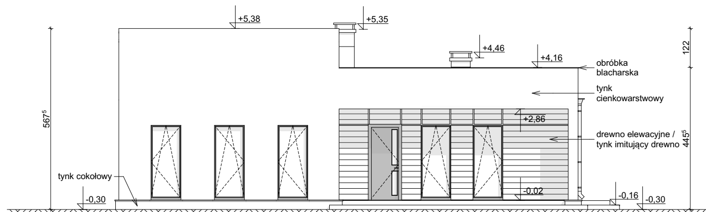
ELEWACJA FRONTOWA
