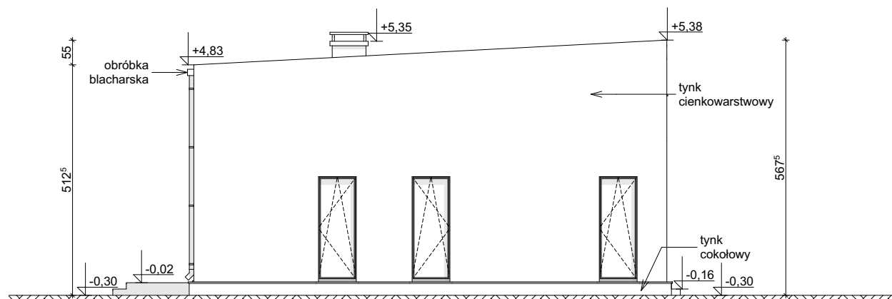
ELEWACJA BOCZNA
