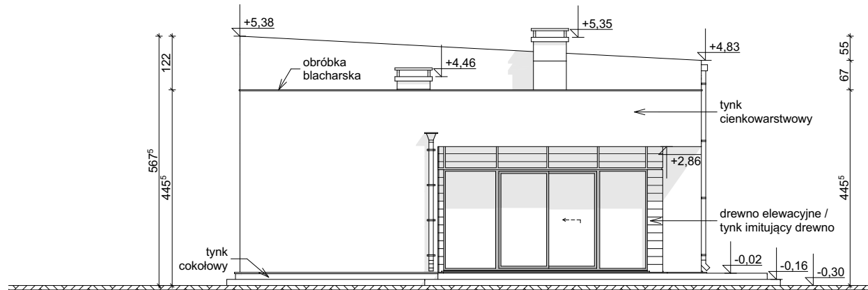
ELEWACJA BOCZNA
