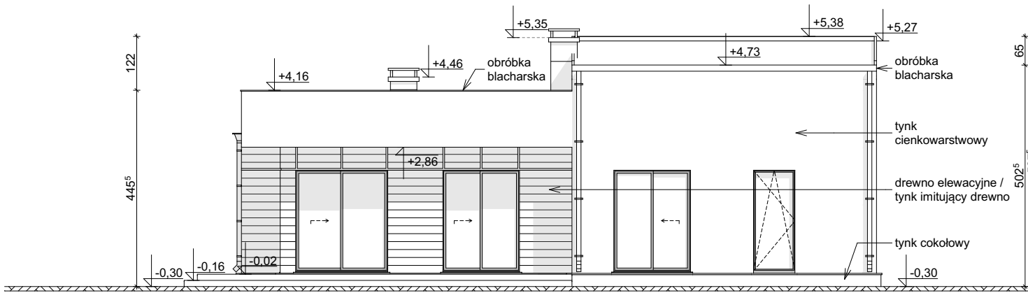
ELEWACJA OGRODOWA
