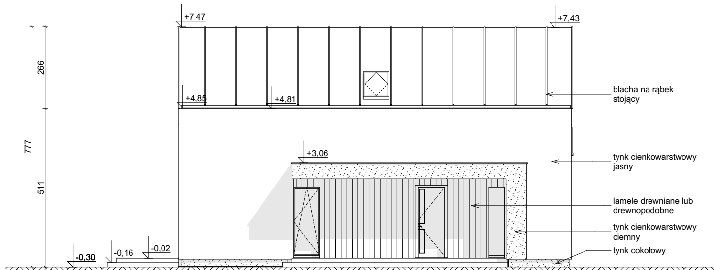
ELEWACJA FRONTOWA
