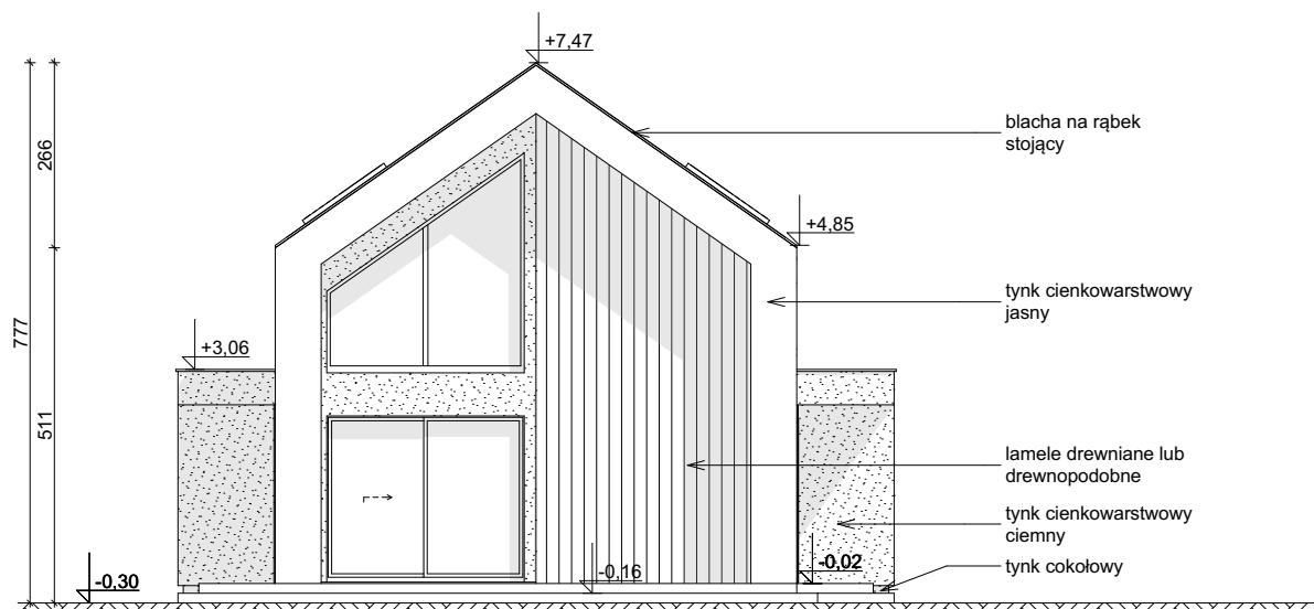
ELEWACJA BOCZNA
