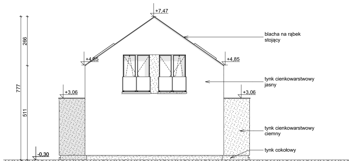
ELEWACJA BOCZNA
