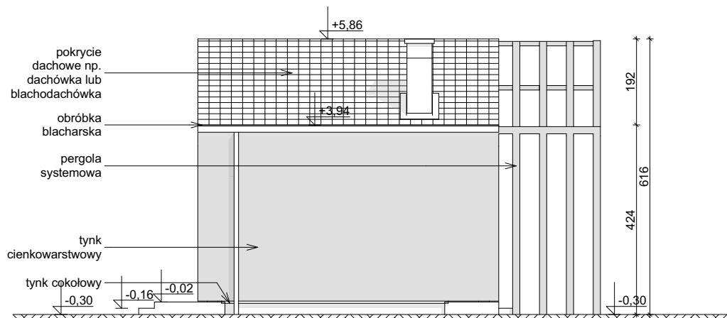
ELEWACJA BOCZNA
