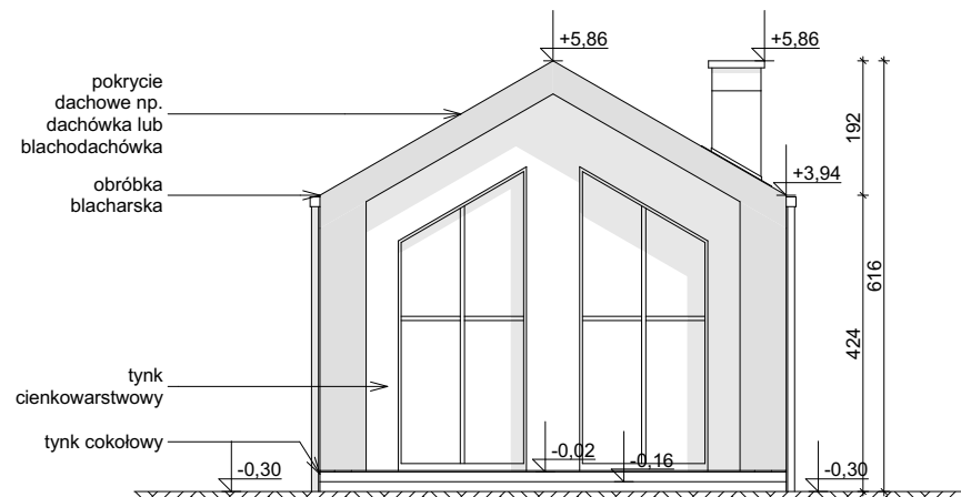
ELEWACJA OGRODOWA
