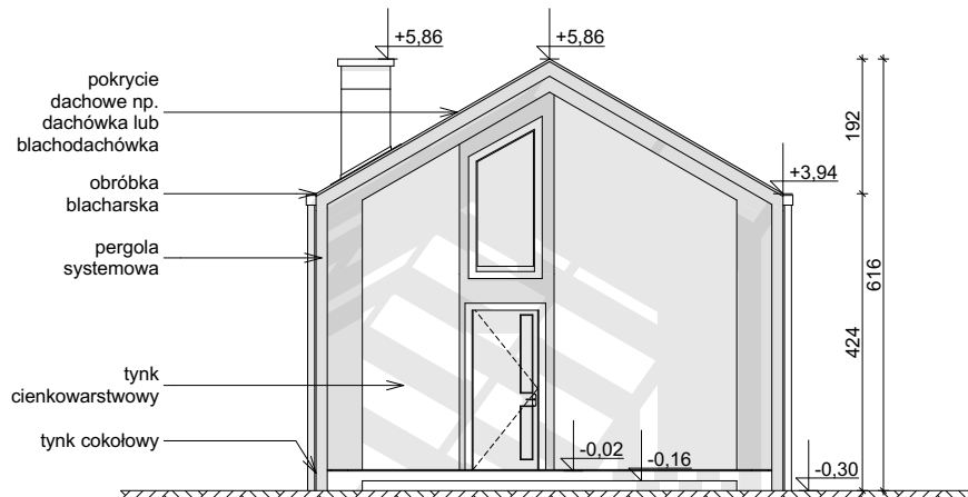
ELEWACJA FRONTOWA
