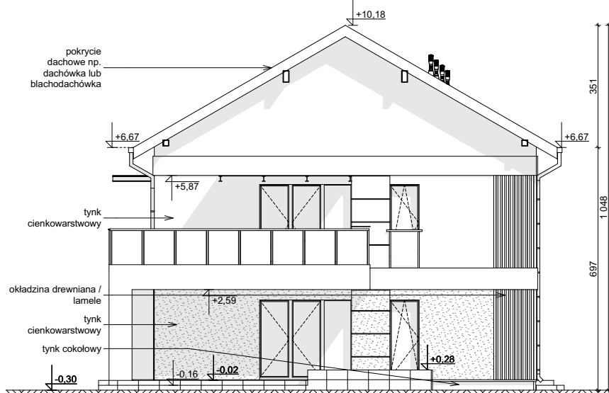
ELEWACJA BOCZNA
