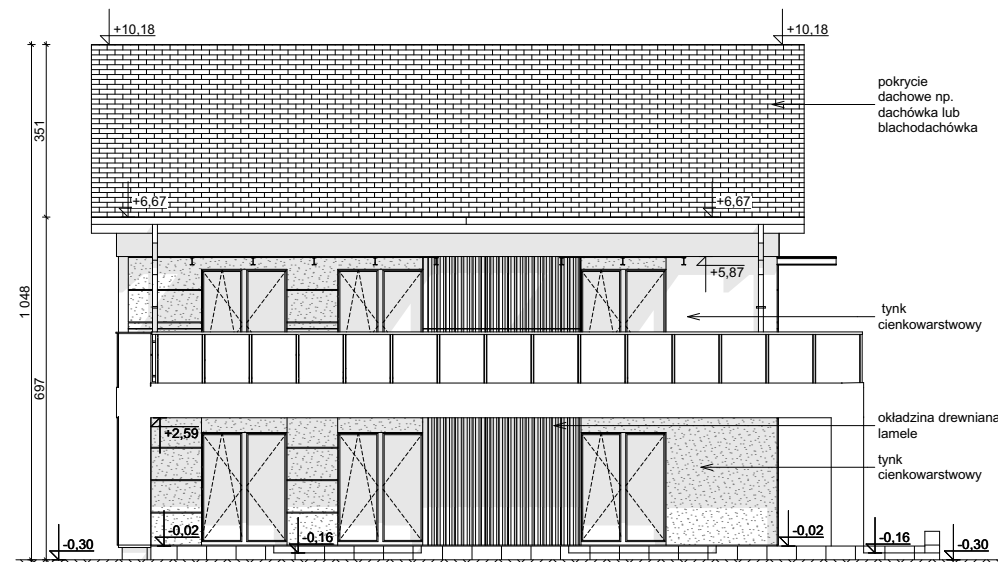
ELEWACJA OGRODOWA
