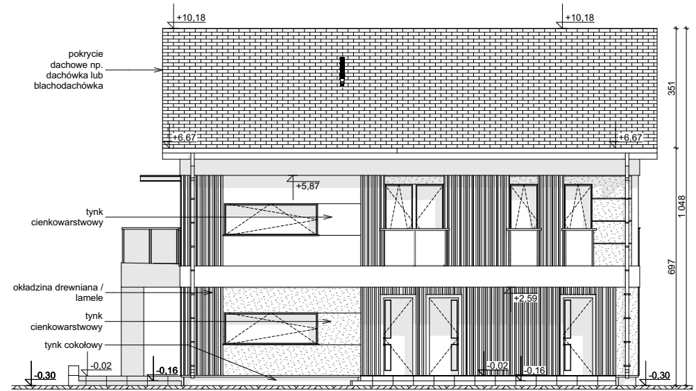
ELEWACJA FRONTOWA
