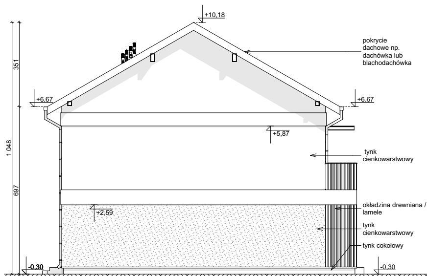
ELEWACJA BOCZNA
