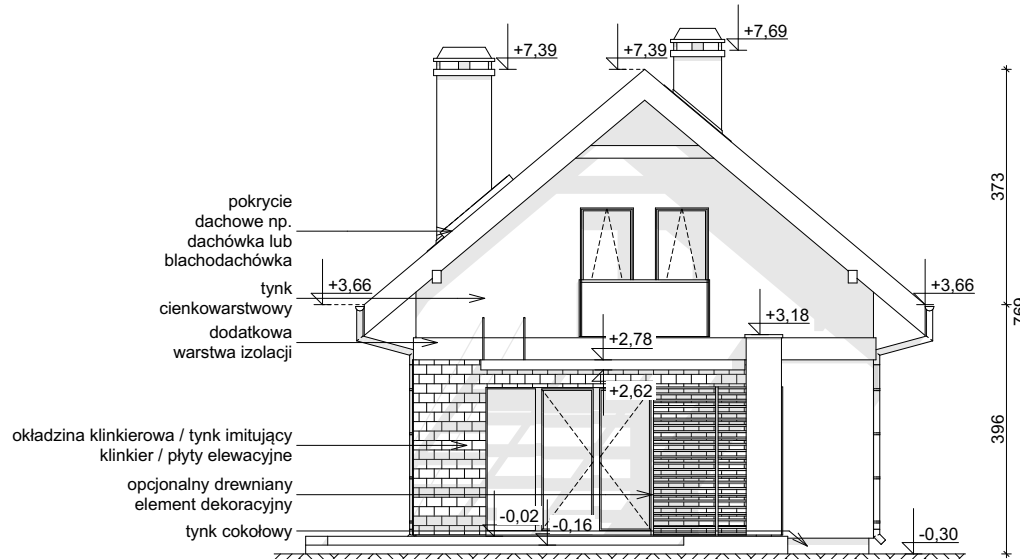
ELEWACJA OGRODOWA
