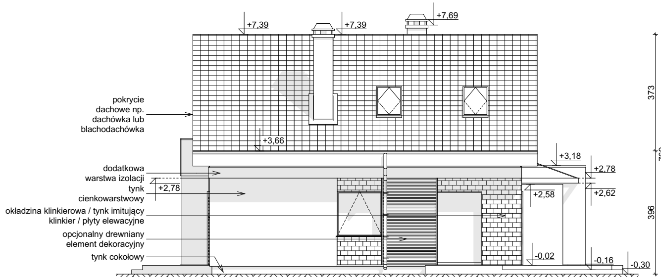
ELEWACJA BOCZNA
