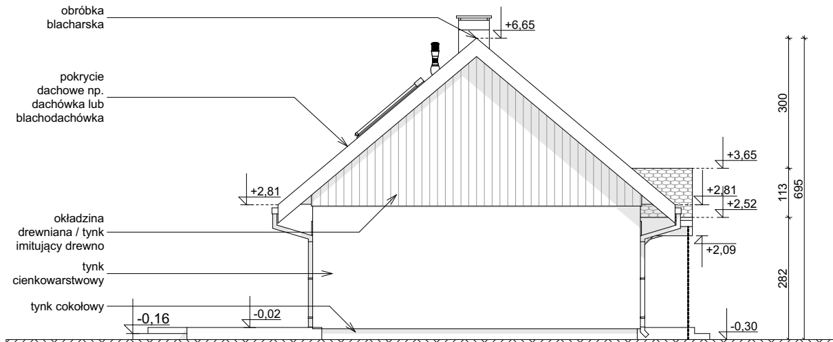
ELEWACJA BOCZNA
