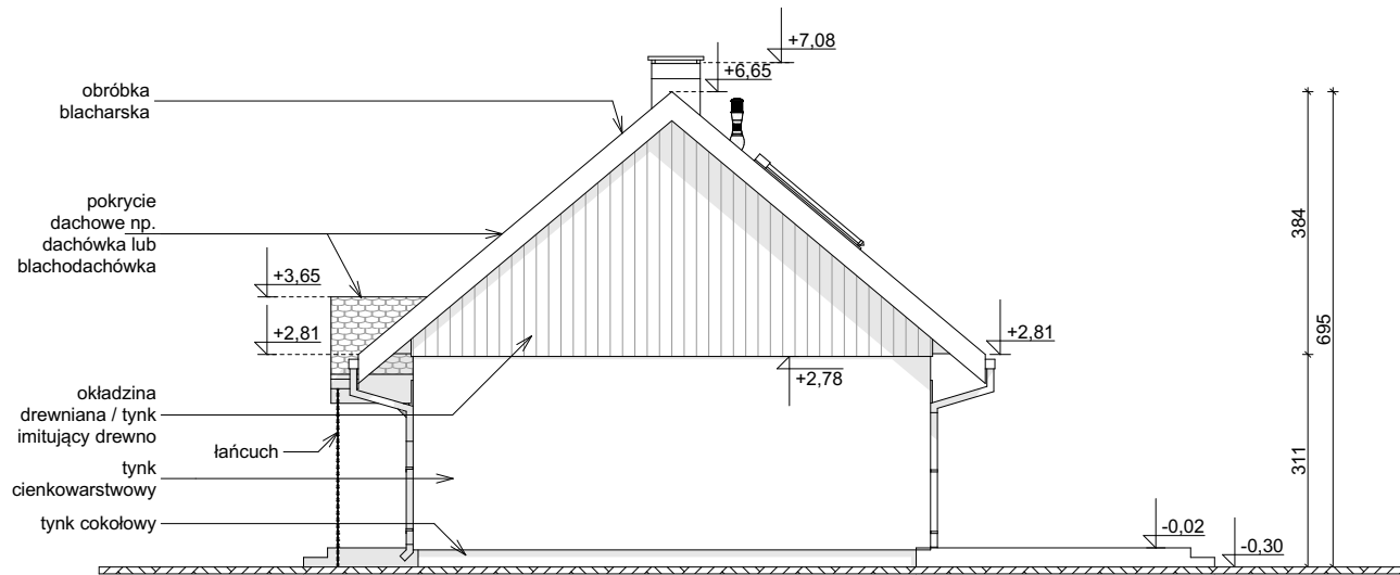
ELEWACJA BOCZNA
