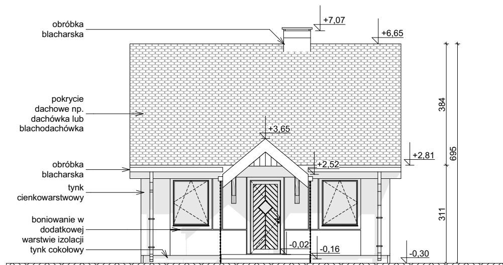
ELEWACJA FRONTOWA
