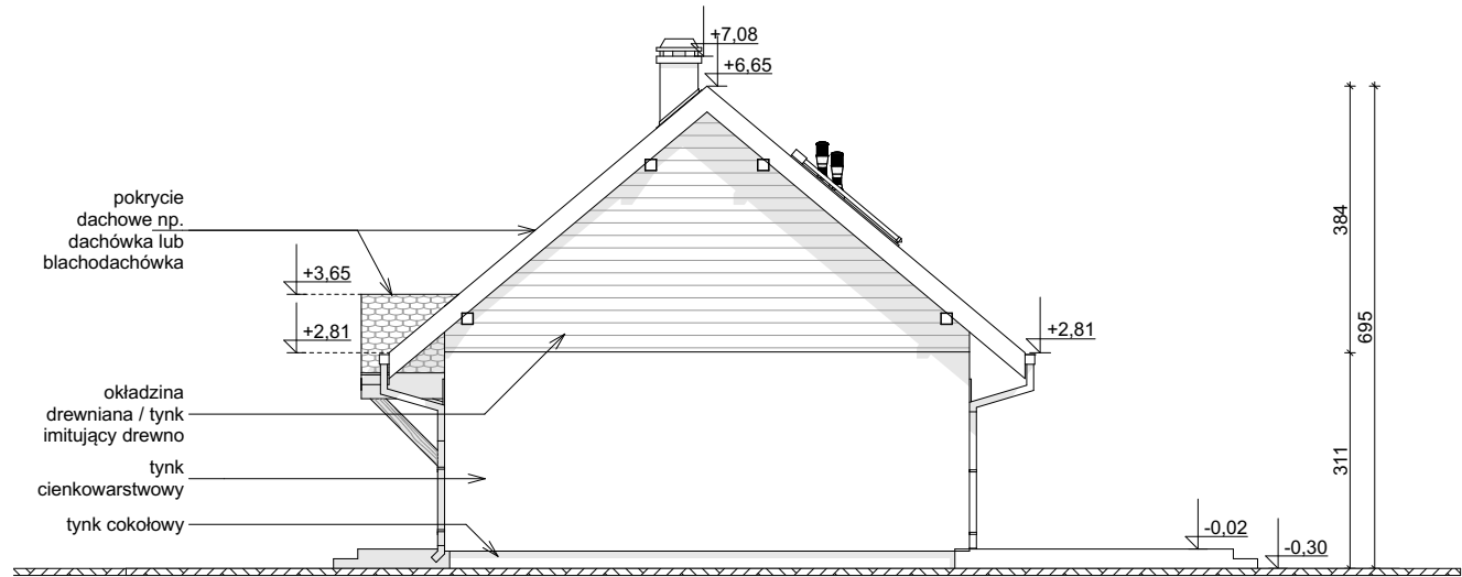
ELEWACJA BOCZNA
