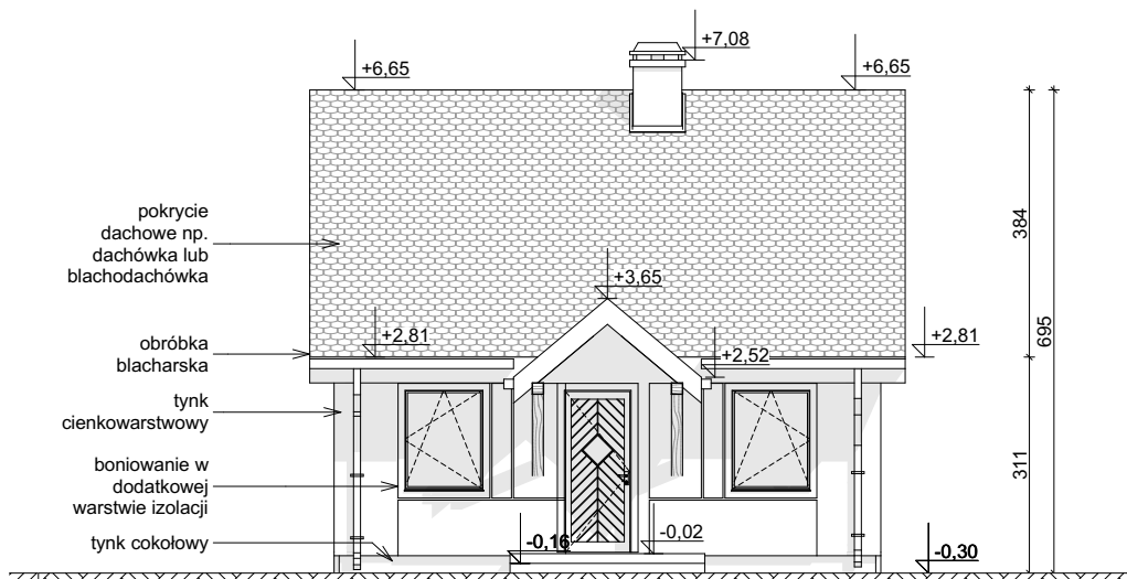
ELEWACJA FRONTOWA
