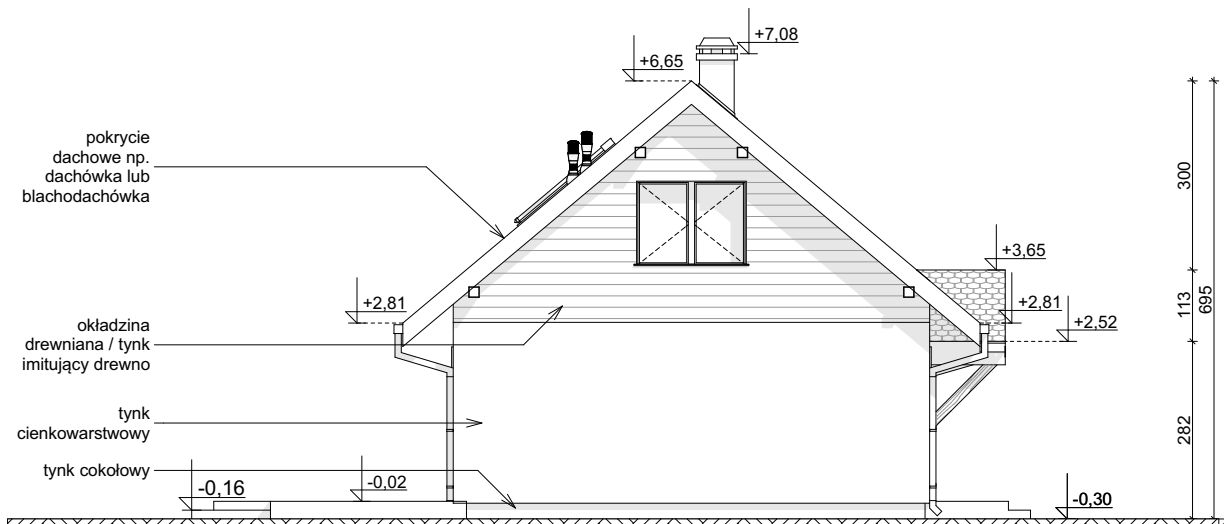
ELEWACJA FRONTOWA
