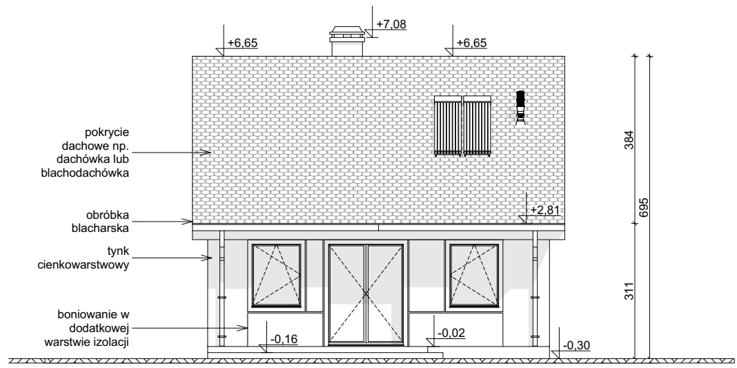
ELEWACJA OGRODOWA
