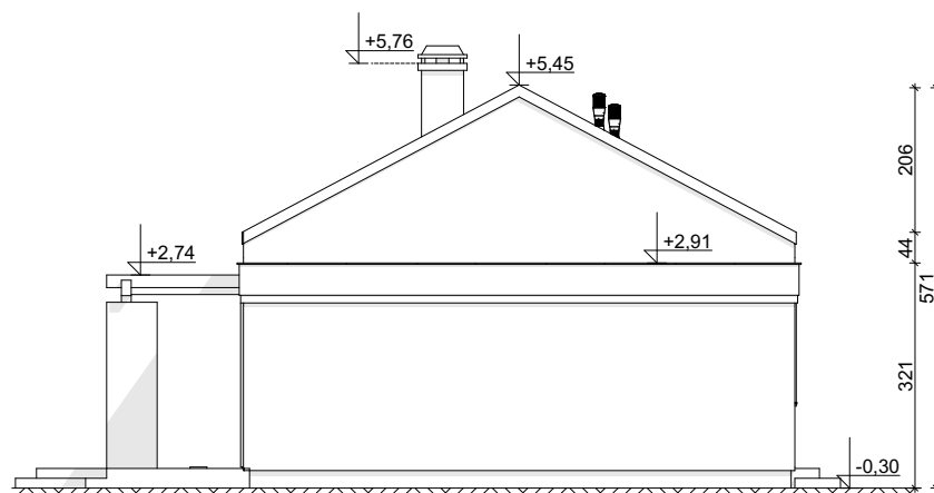
ELEWACJA BOCZNA
