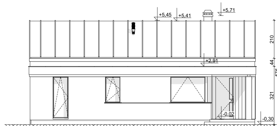
ELEWACJA FRONTOWA
