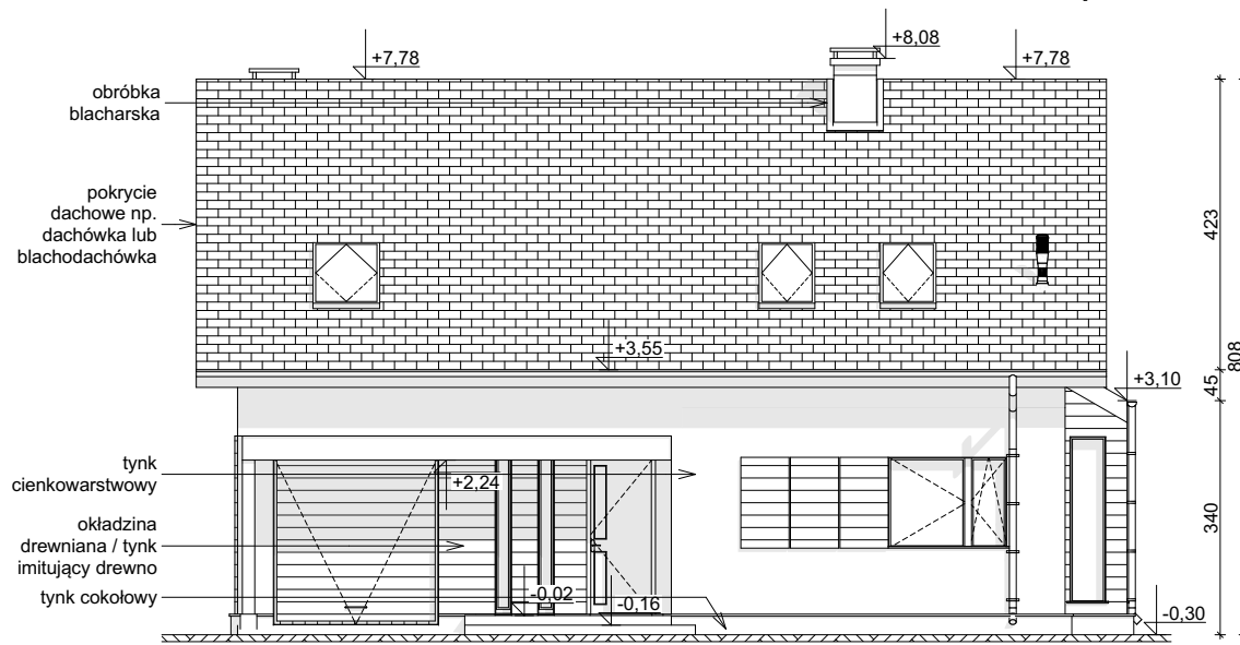
ELEWACJA FRONTOWA
