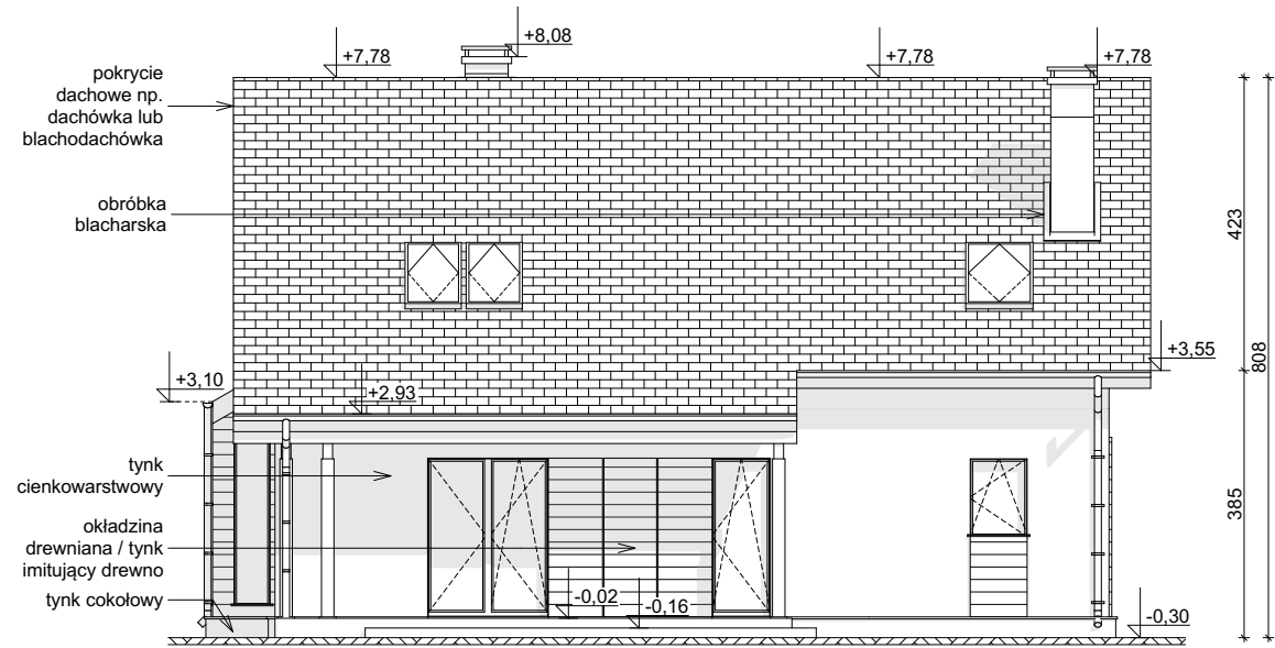
ELEWACJA OGRODOWA
