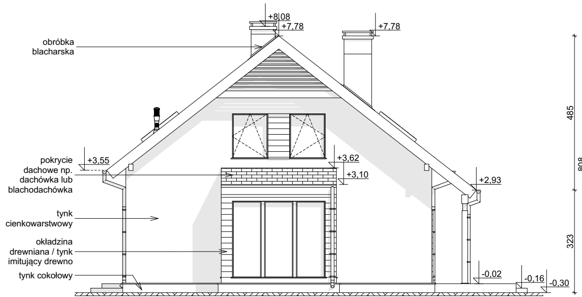
ELEWACJA BOCZNA
