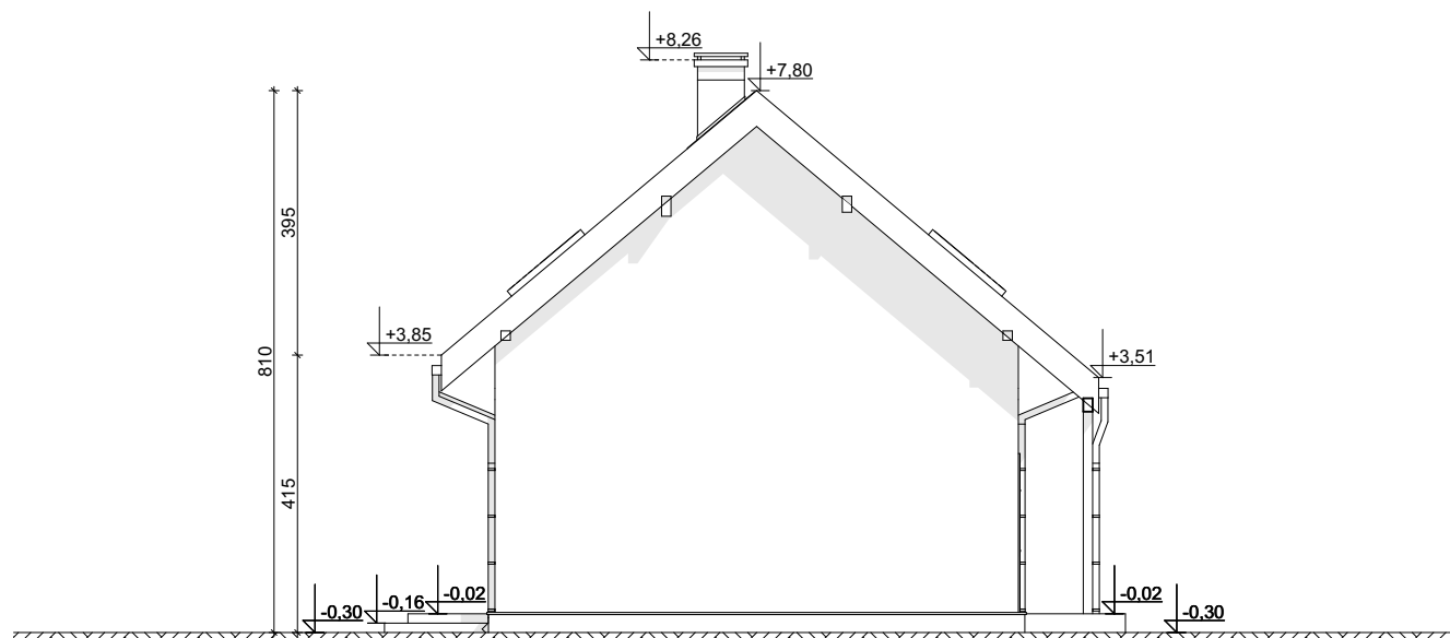
ELEWACJA BOCZNA
