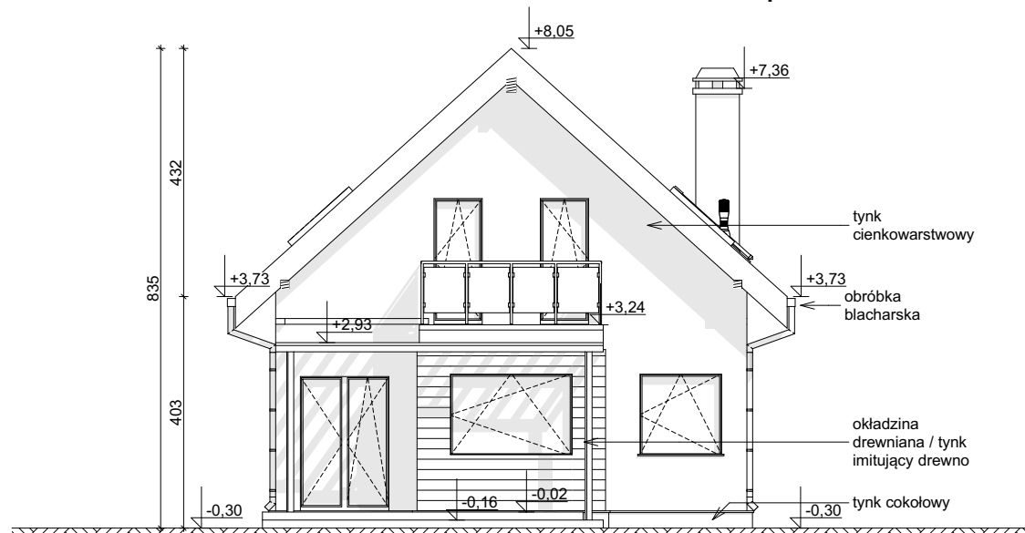
ELEWACJA OGRODOWA
