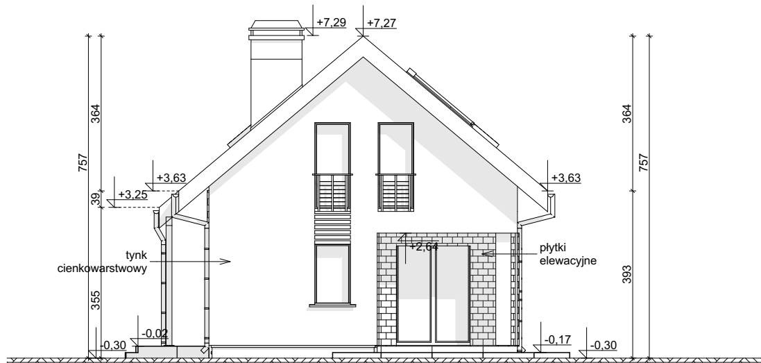
ELEWACJA BOCZNA
