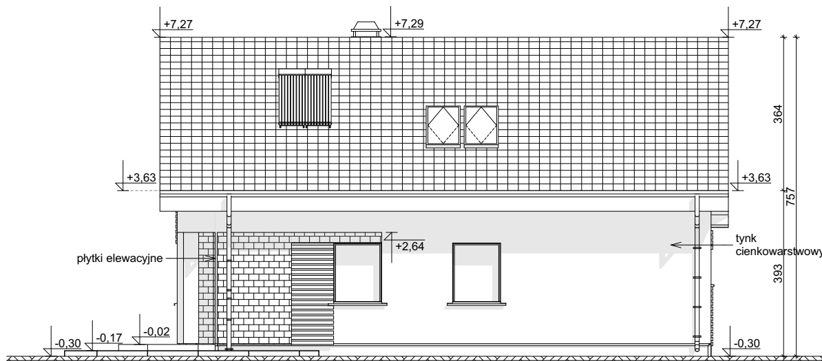
ELEWACJA OGRODOWA
