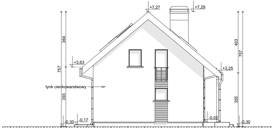
ELEWACJA BOCZNA
