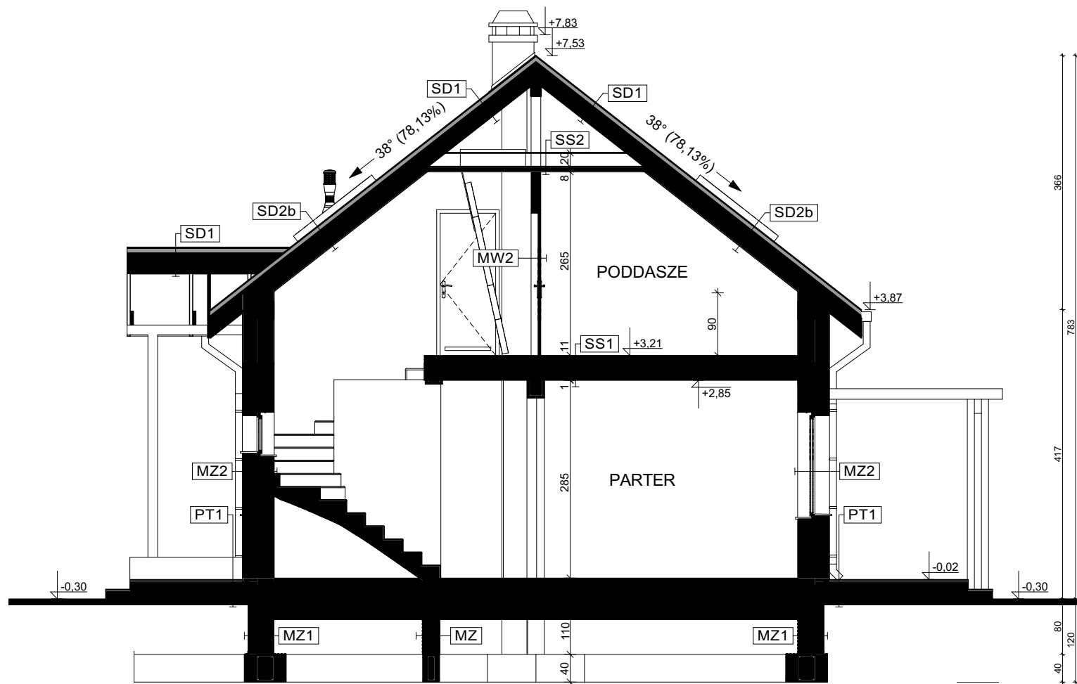
PRZEKRÓJ B-B
