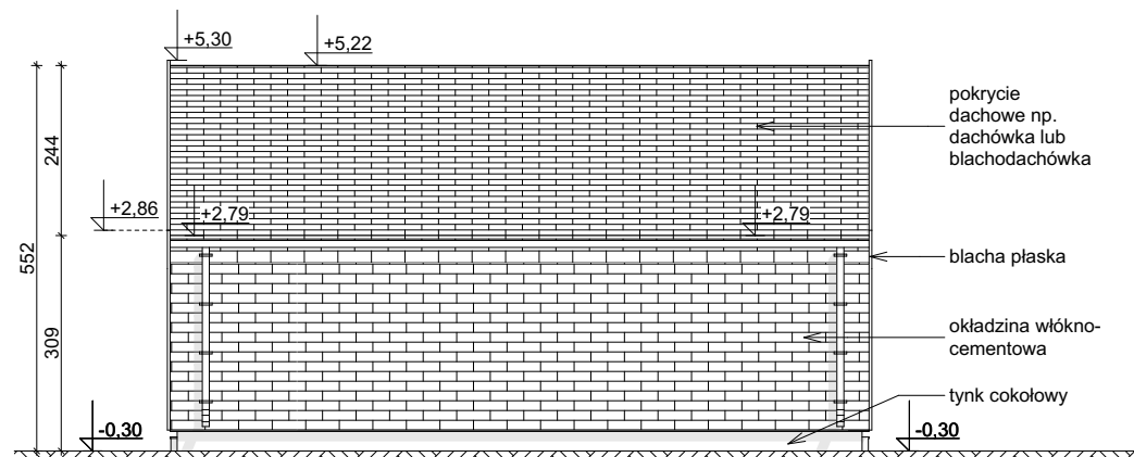
ELEWACJA OGRODOWA
