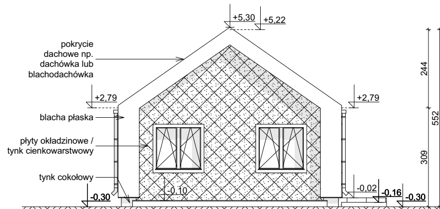
ELEWACJA BOCZNA
