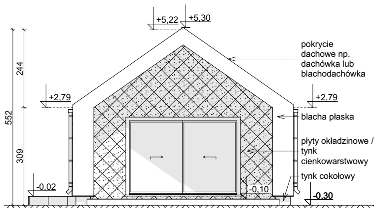
ELEWACJA BOCZNA
