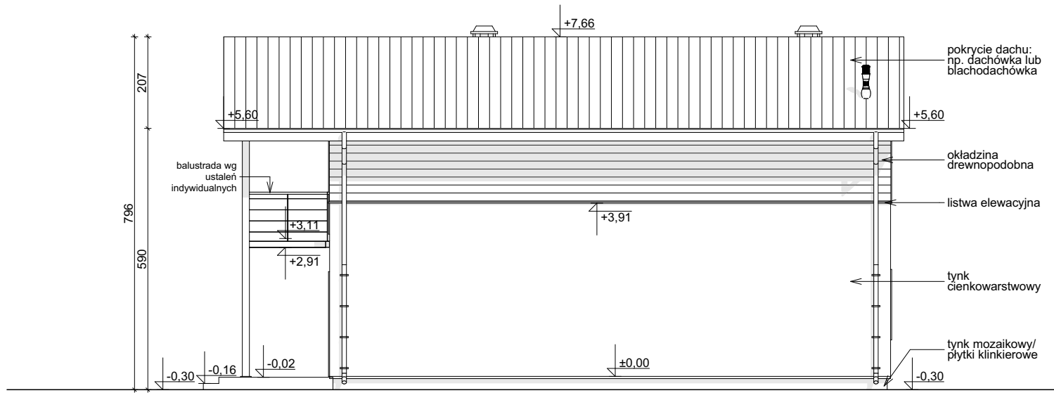
ELEWACJA BOCZNA
