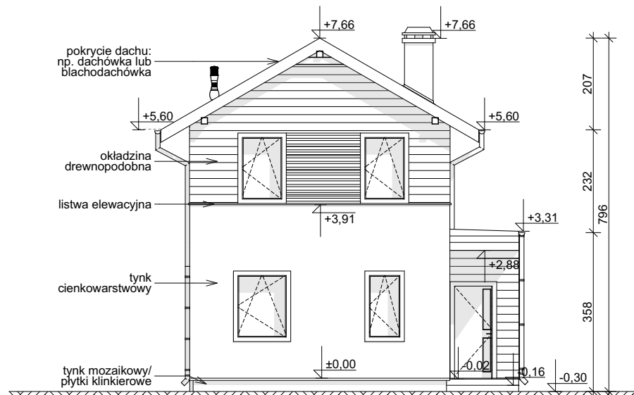
ELEWACJA FRONTOWA
