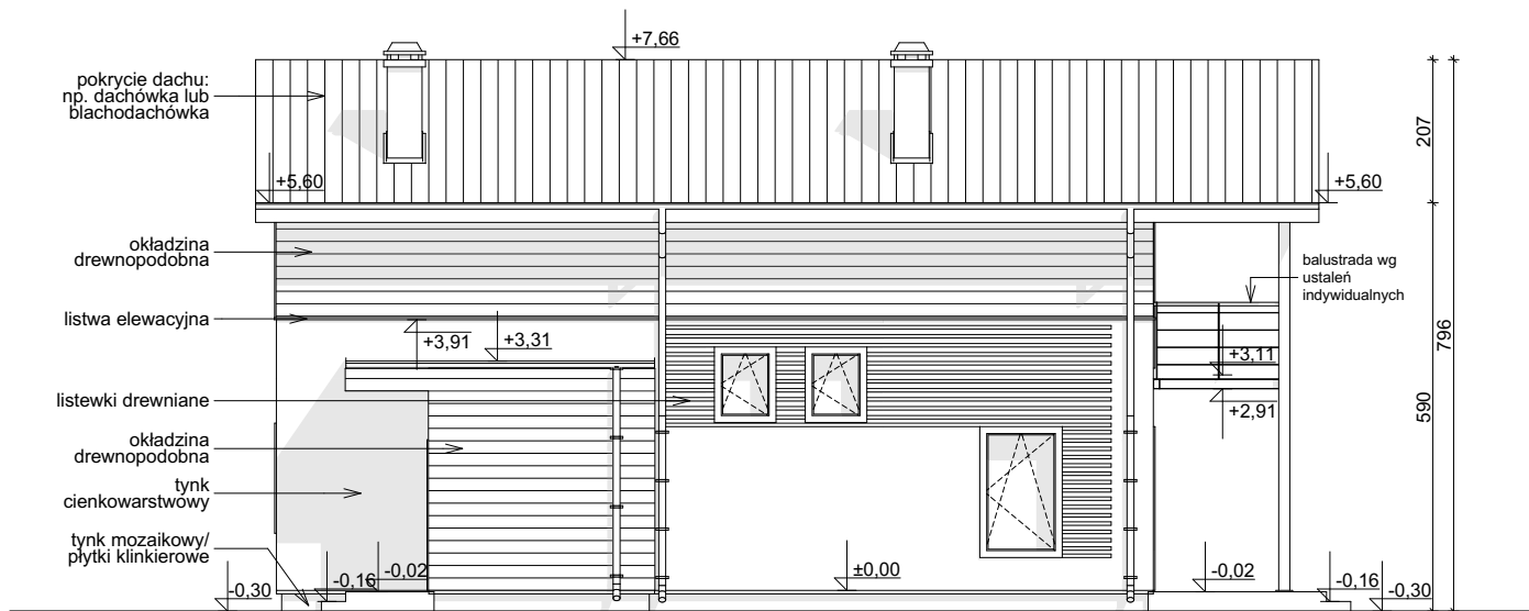
ELEWACJA BOCZNA
