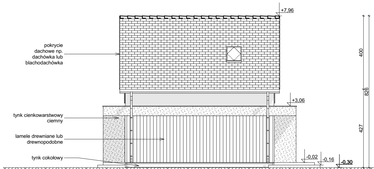
ELEVACJA BOCZNA
