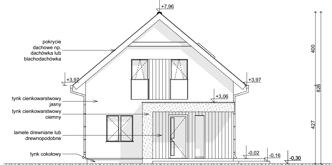
ELEWACJA FRONTOWA
