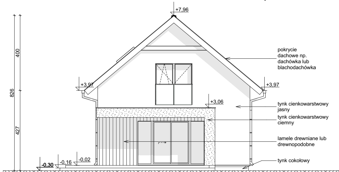
ELEVACJA OGRODOWA
