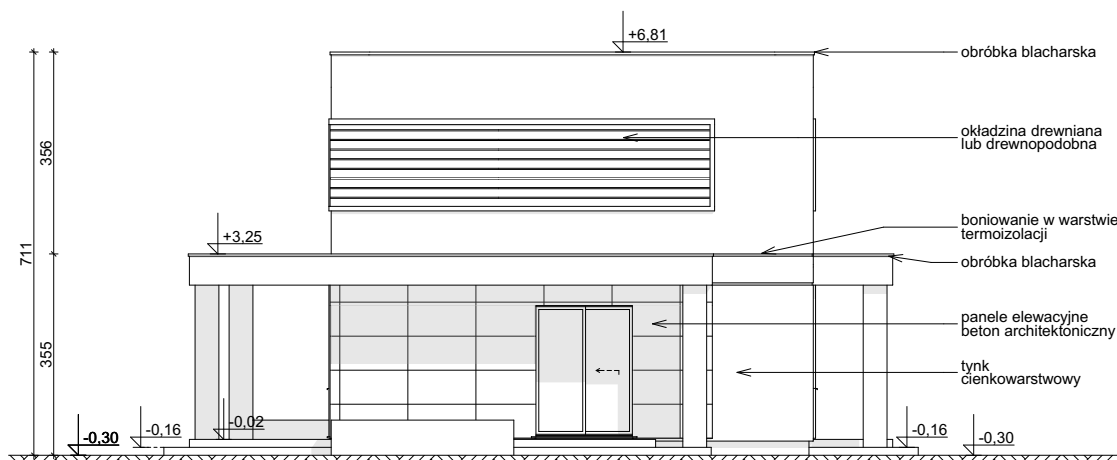
ELEWACJA BOCZNA
