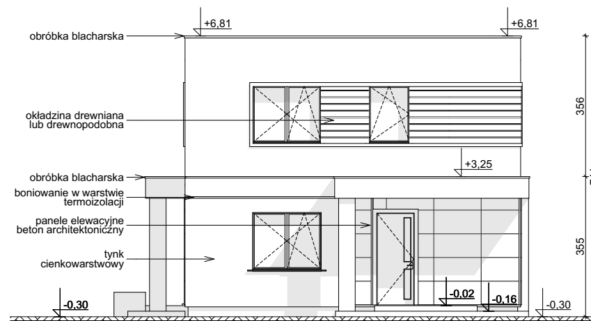
ELEWACJA FRONTOWA
