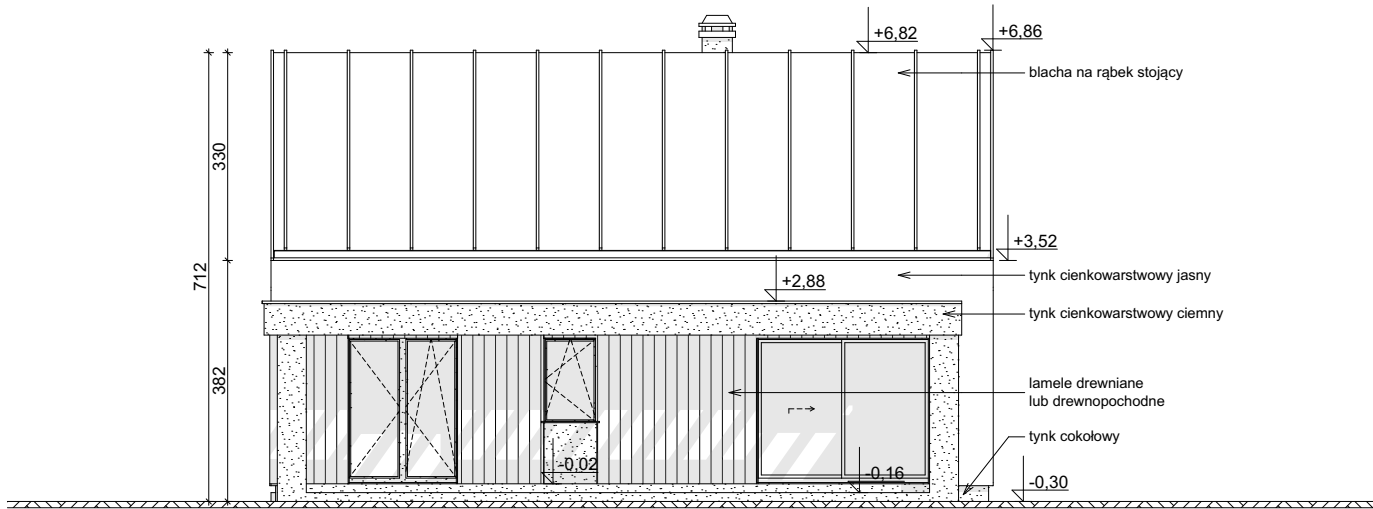
ELEVACJA OGRODOWA
