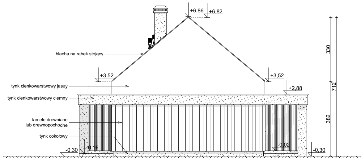
ELEVACJA BOCZNA
