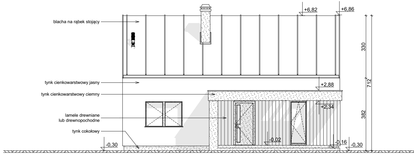
ELEWACJA FRONTOWA
