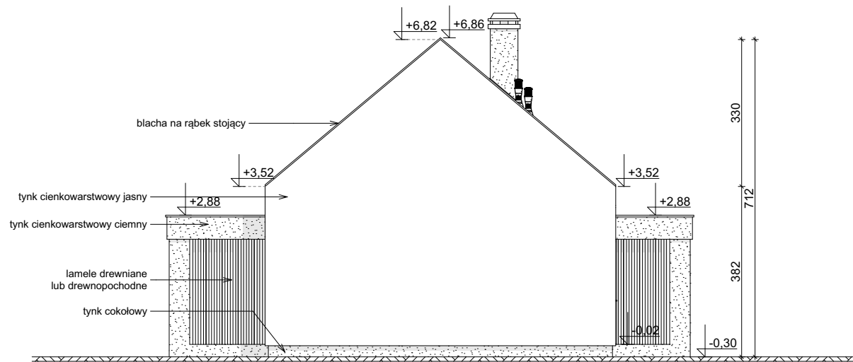
ELEWACJA BOCZNA
