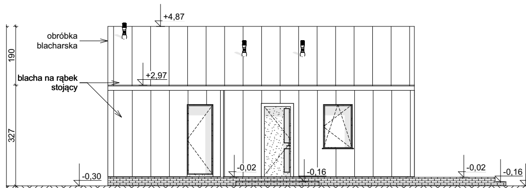
ELEWACJA FRONTOWA
