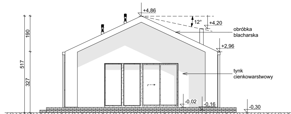
ELEWACJA BOCZNA
