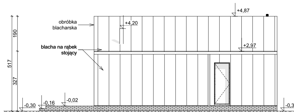
ELEWACJA OGRODOWA
