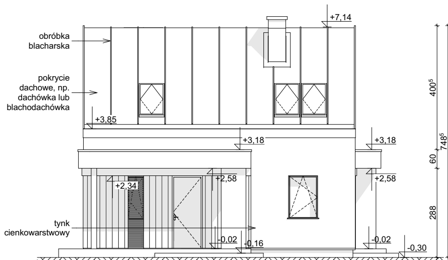
ELEWACJA FRONTOWA
