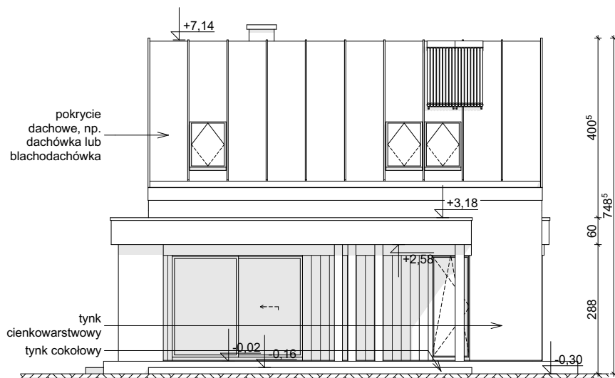
ELEWACJA OGRODOWA
