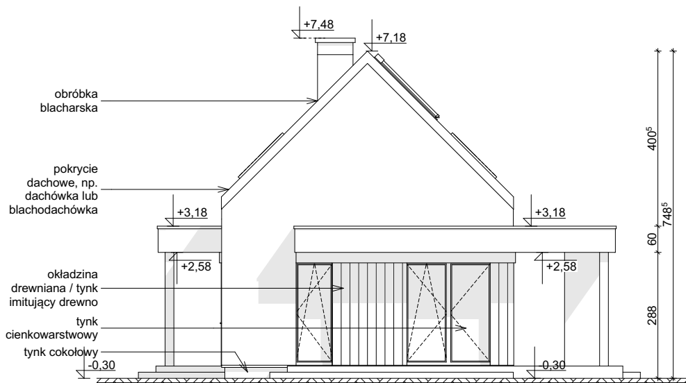
ELEWACJA BOCZNA
