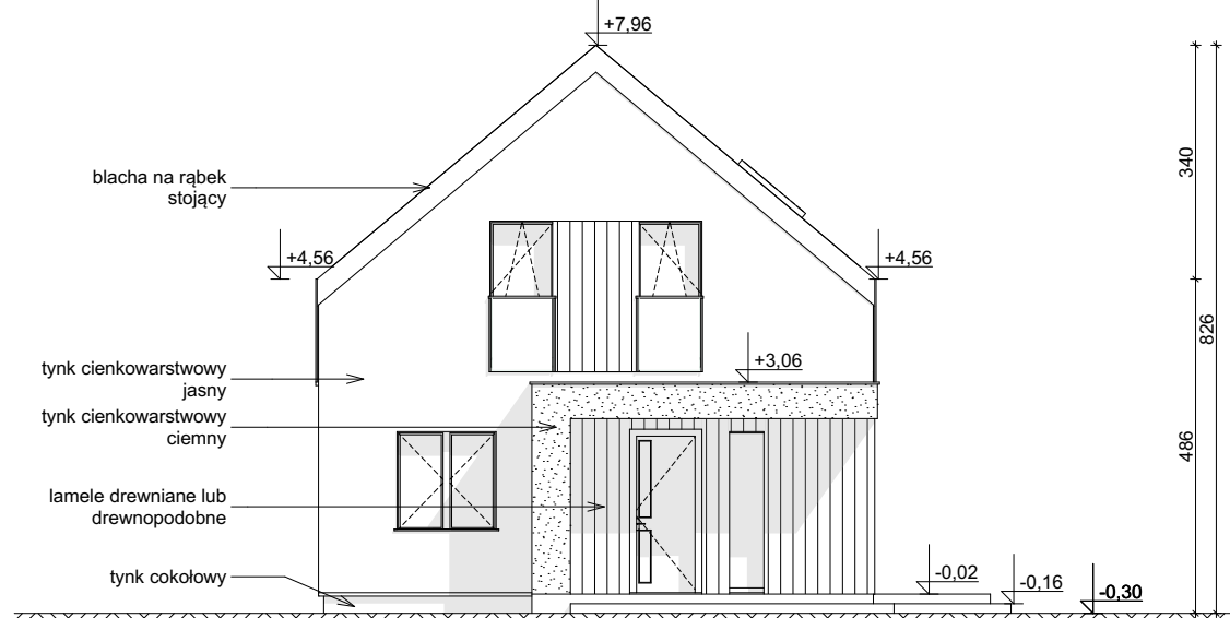
ELEWACJA FRONTOWA
