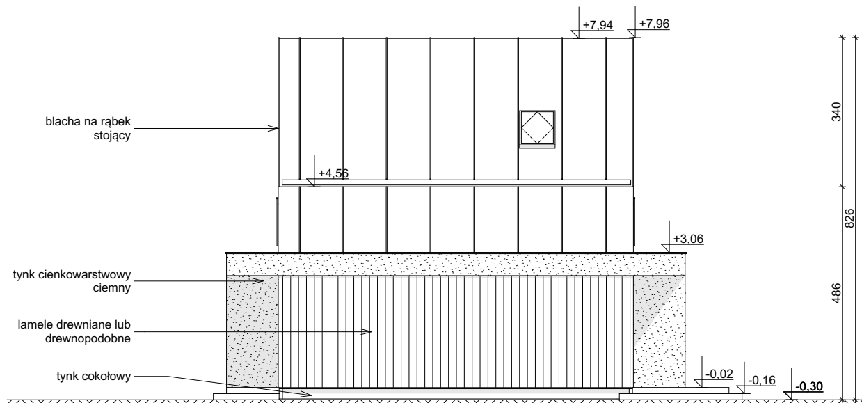
ELEWACJA BOCZNA
