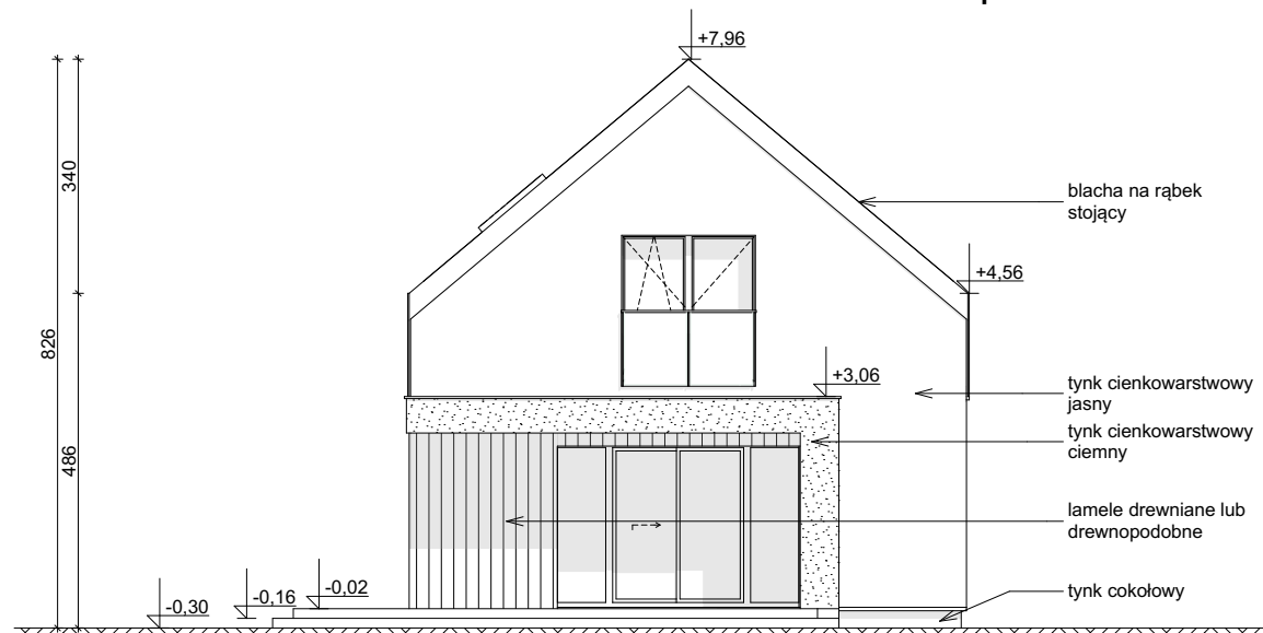
ELEWACJA OGRODOWA
