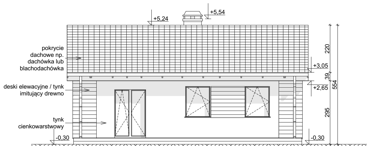
ELEWACJA BOCZNA
