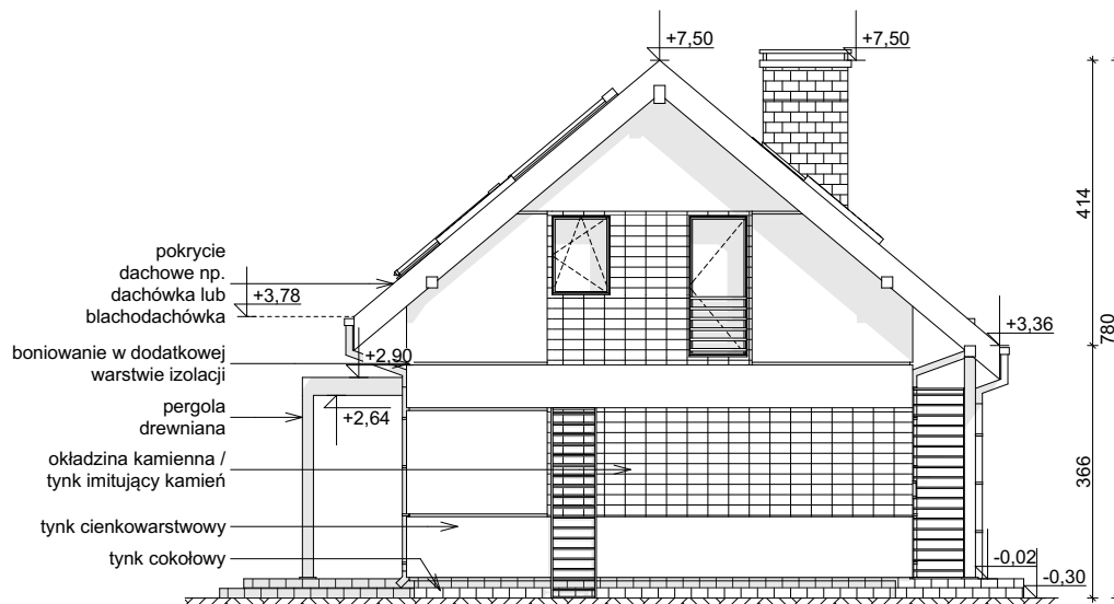
ELEWACJA BOCZNA
