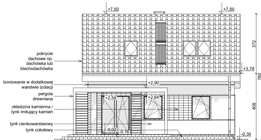
ELEWACJA OGRODOWA
