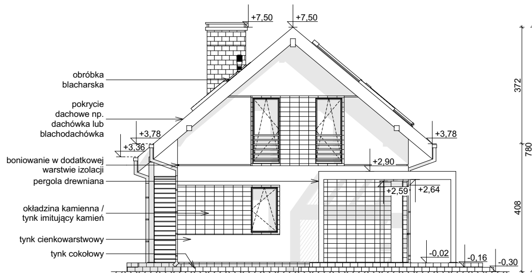
ELEWACJA BOCZNA
