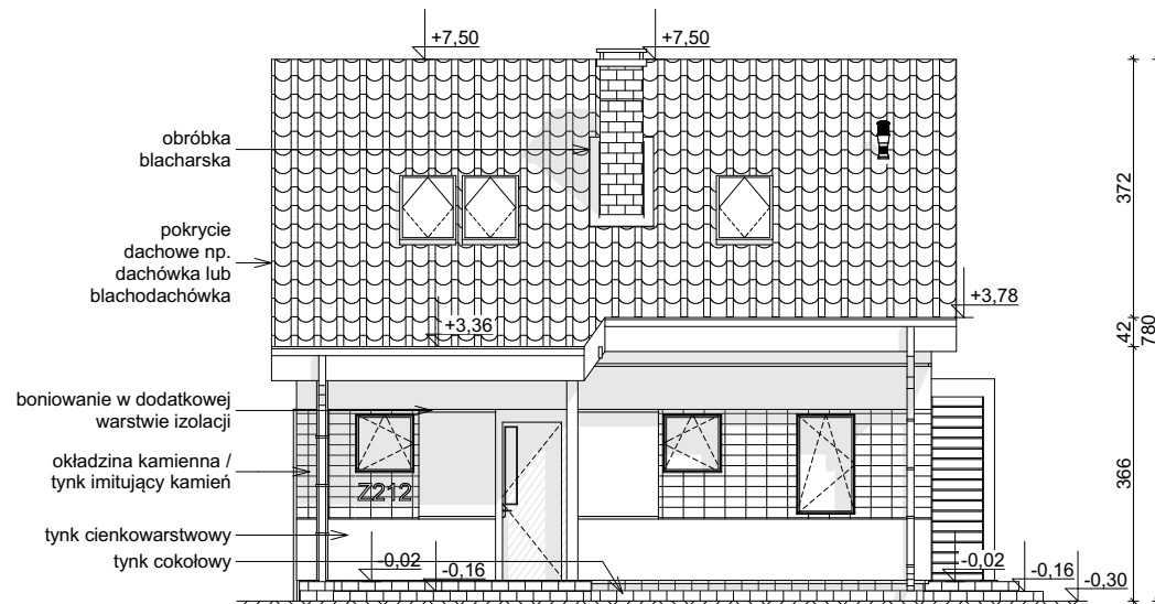
ELEWACJA FRONTOWA
