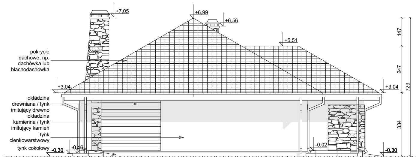
ELEWACJA BOCZNA
