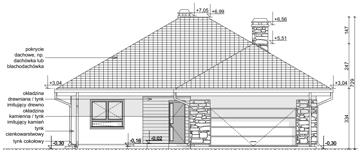
ELEWACJA FRONTOWA
