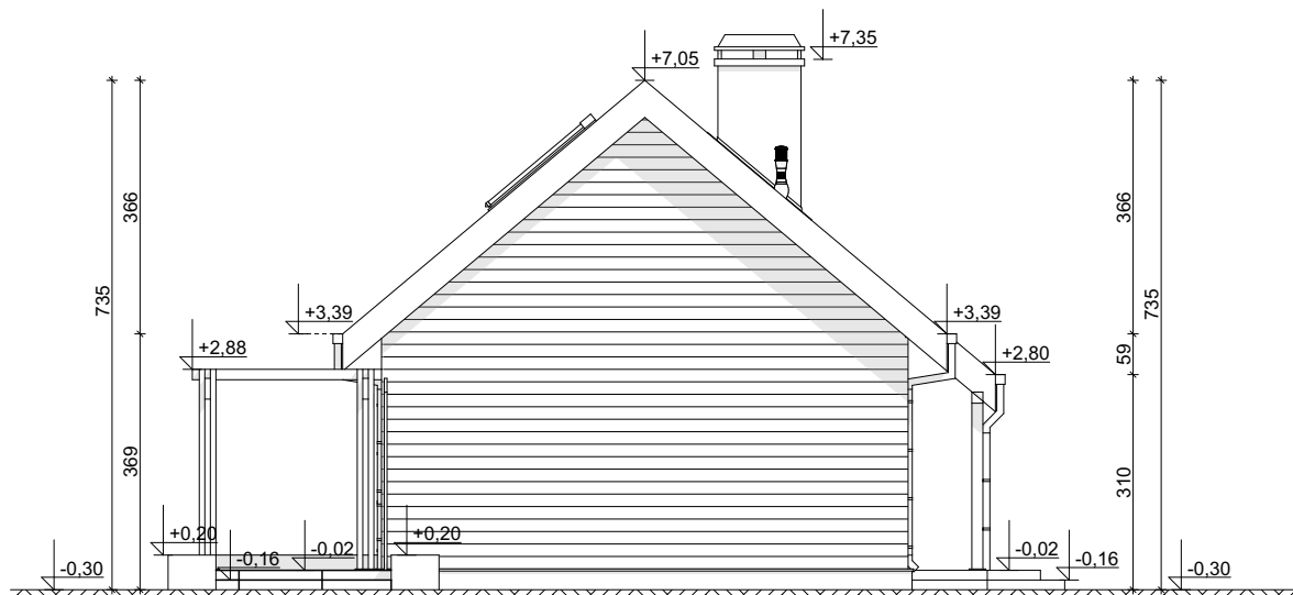
ELEWACJA BOCZNA
