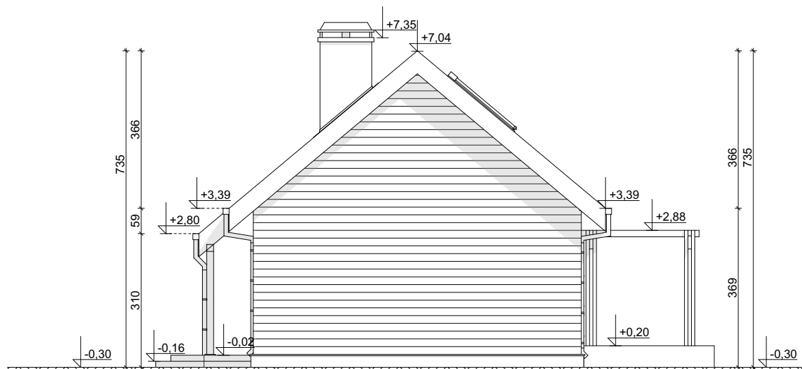
ELEWACJA BOCZNA
