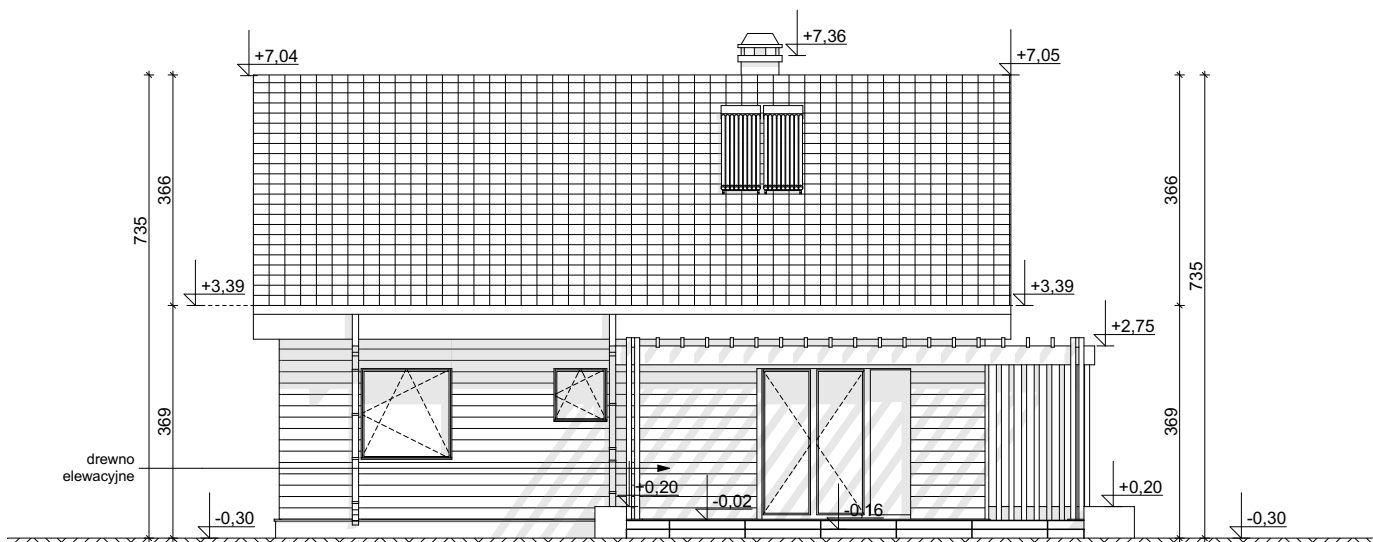
ELEWACJA OGRODOWA
