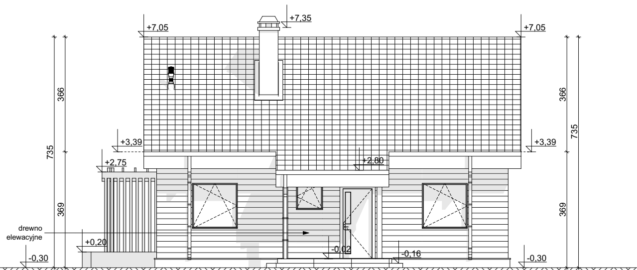
ELEWACJA FRONTOWA
