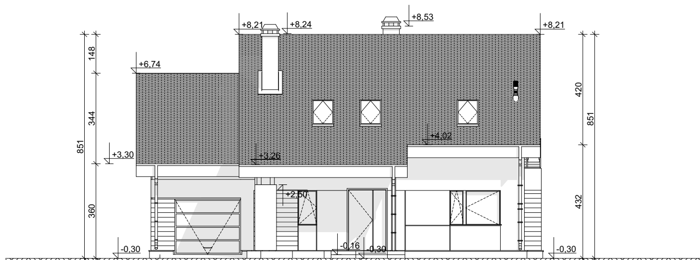
ELEWACJA FRONTOWA
