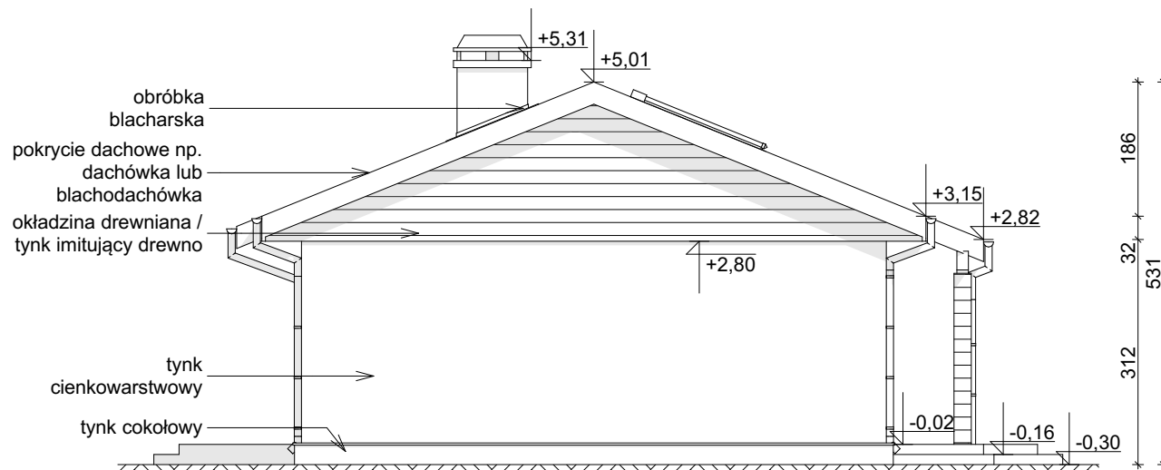
ELEWACJA BOCZNA
