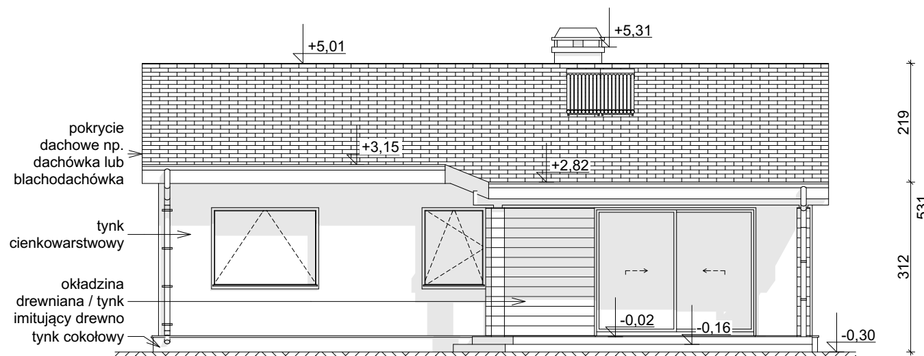
ELEWACJA OGRODOWA
