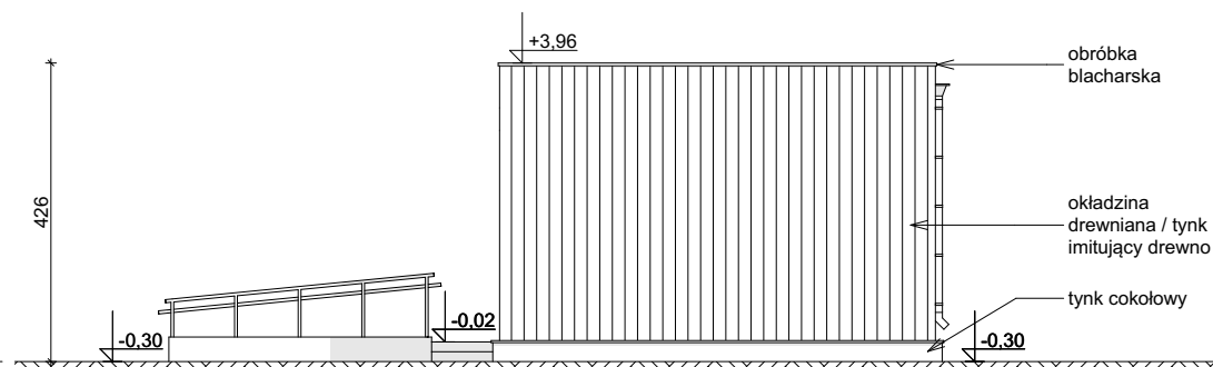
ELEWACJA BOCZNA
