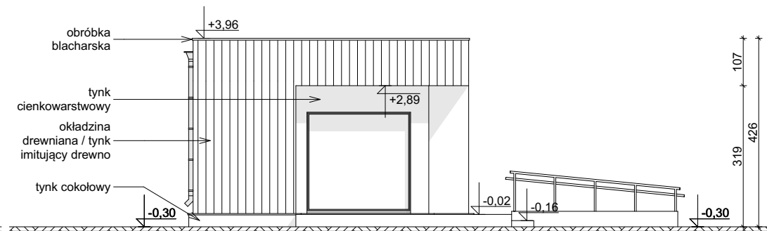
ELEWACJA BOCZNA
