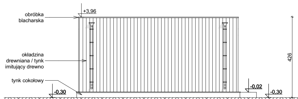
ELEWACJA OGRODOWA
