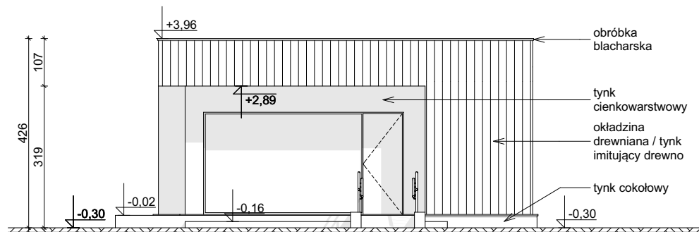
ELEWACJA FRONTOWA
