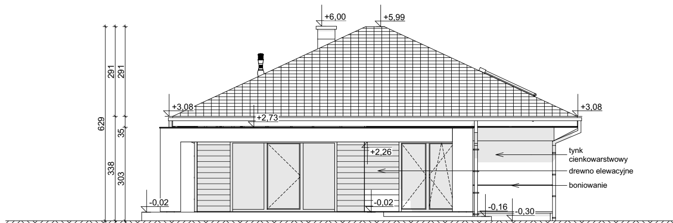
ELEWACJA OGRODOWA
