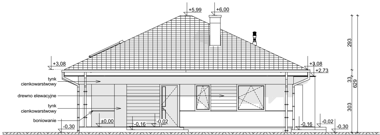
ELEWACJA FRONTOWA
