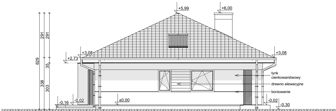
ELEWACJA BOCZNA
