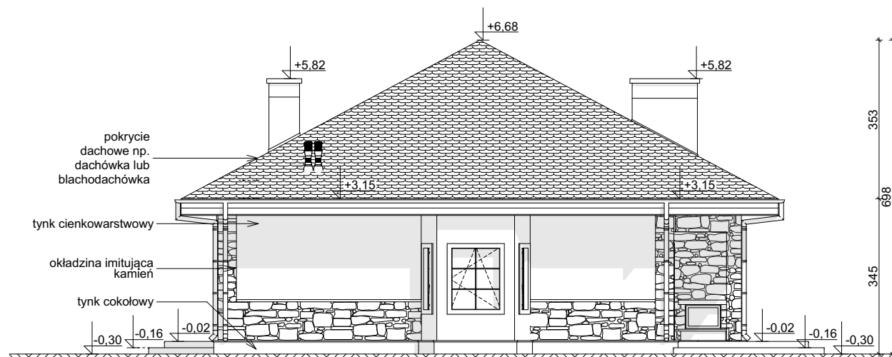
ELEWACJA BOCZNA
