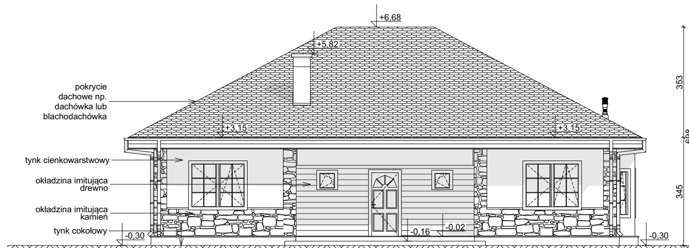
ELEWACJA FRONTOWA
