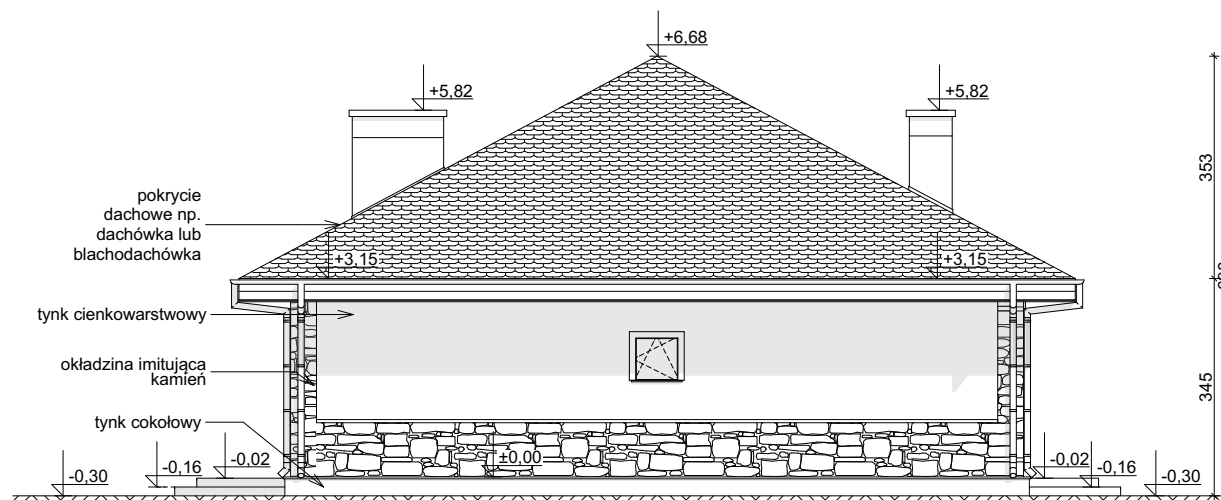
ELEWACJA BOCZNA
