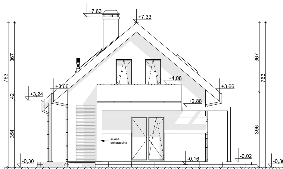
ELEVACJA BOCZNA
