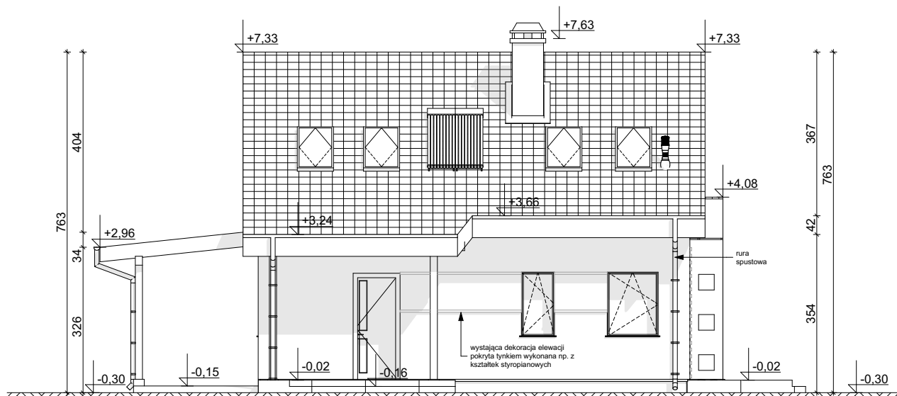
ELEWACJA FRONTOWA
