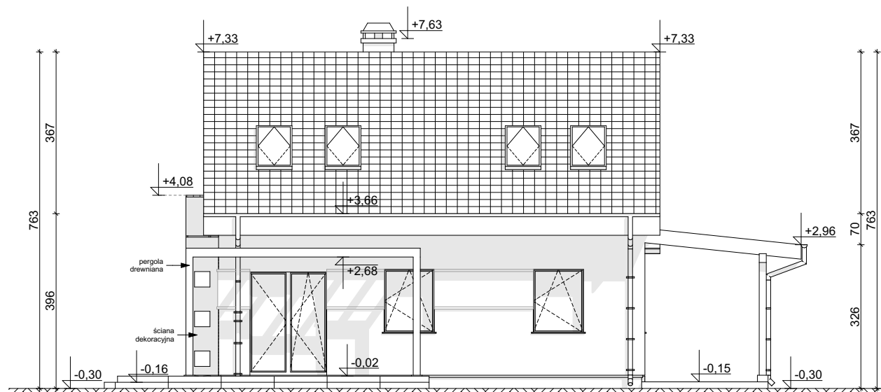
ELEVACJA OGRODOWA
