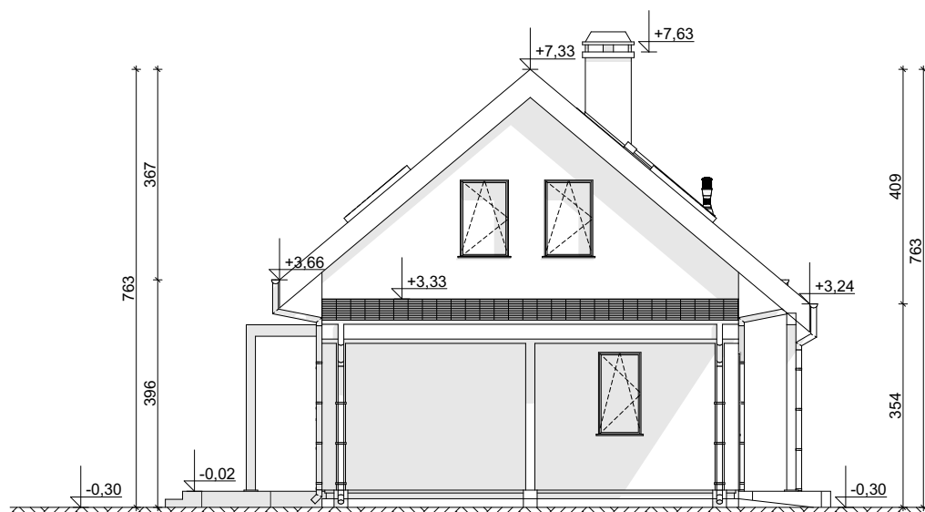
ELEWACJA BOCZNA
