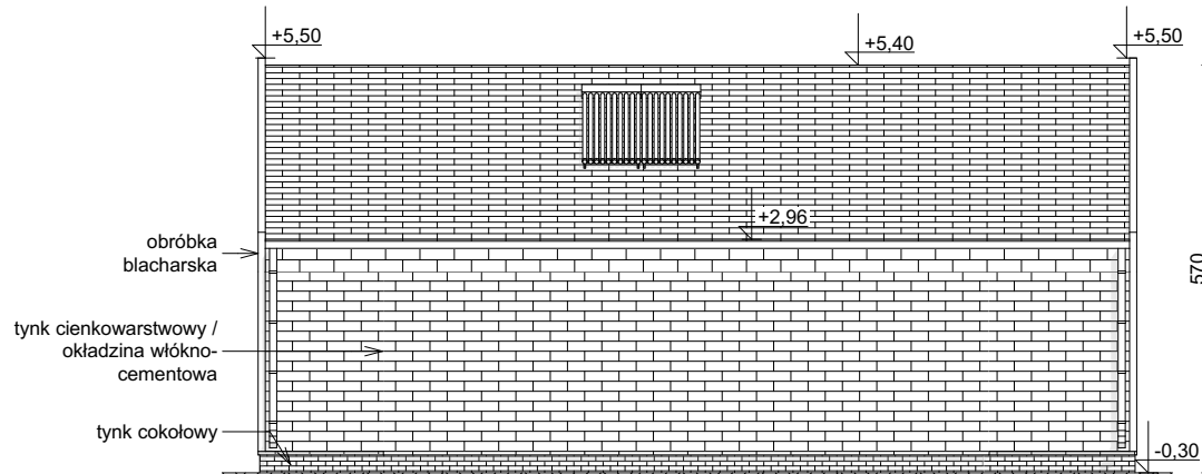
ELEWACJA BOCZNA
