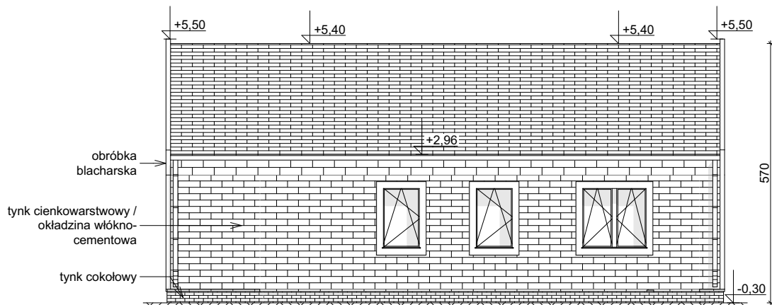
ELEWACJA BOCZNA
