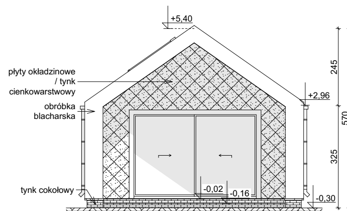
ELEWACJA OGRODOWA
