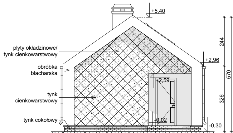
ELEWACJA FRONTOWA
