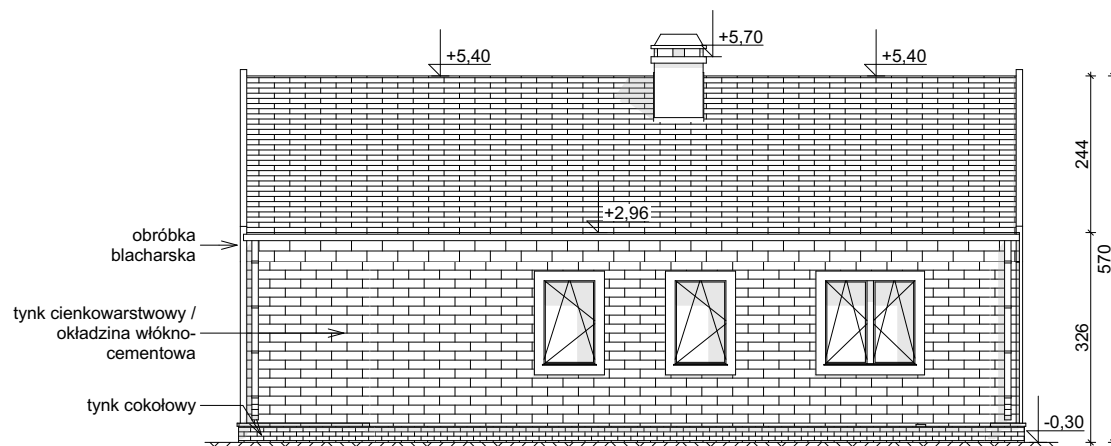
ELEWACJA BOCZNA
