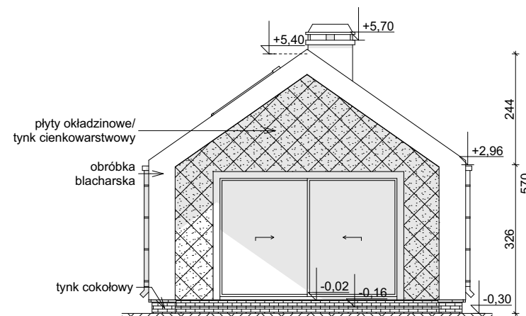
ELEWACJA OGRODOWA
