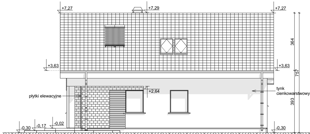
ELEWACJA OGRODOWA
