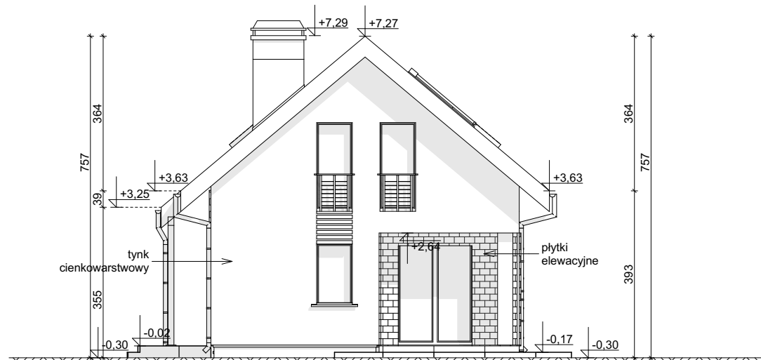
ELEWACJA BOCZNA
