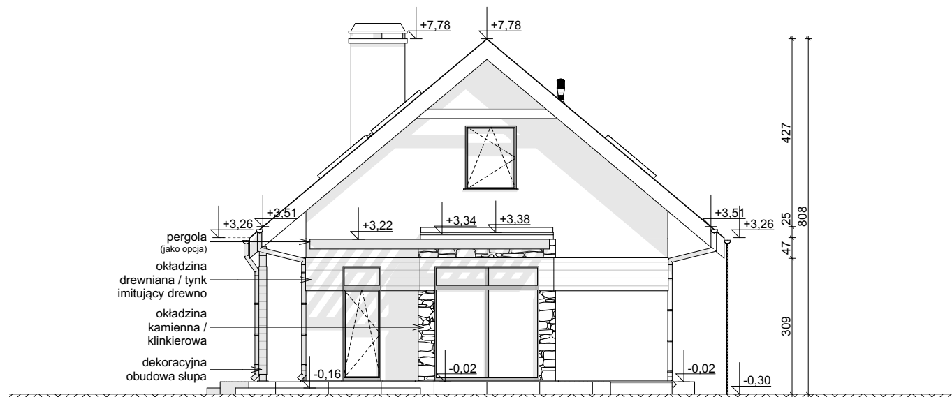
ELEWACJA BOCZNA
