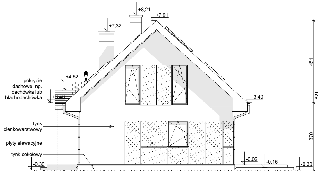
ELEVACJA BOCZNA
