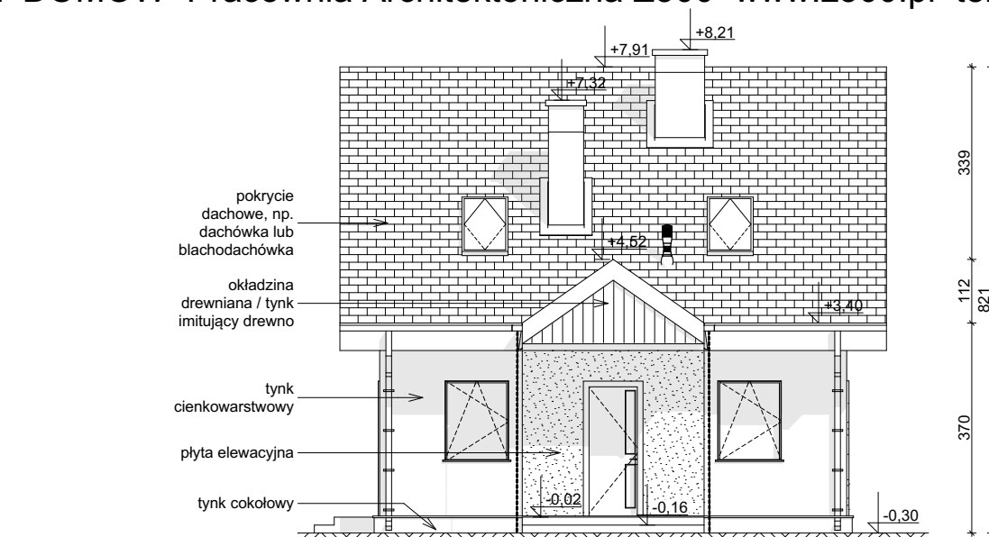
ELEWACJA FRONTOWA
