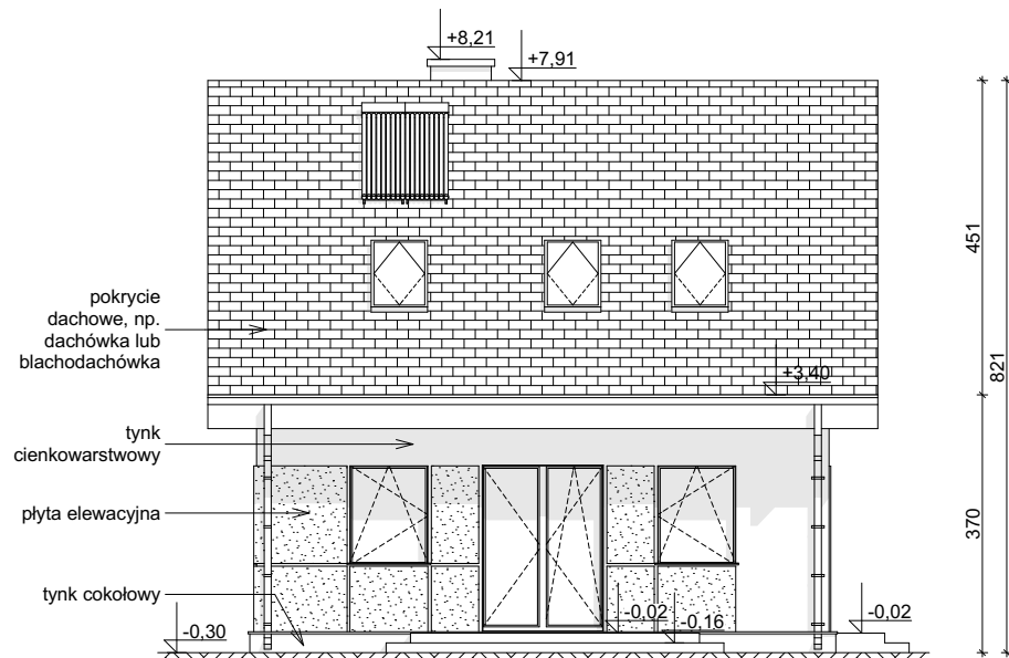
ELEVACJA OGRODOWA
