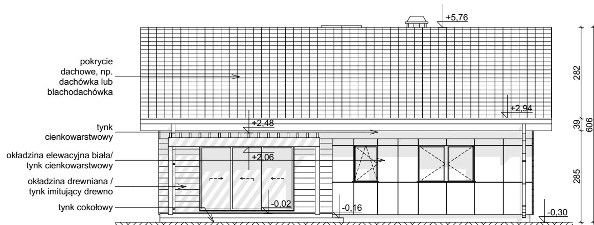
ELEWACJA OGRODOWA
