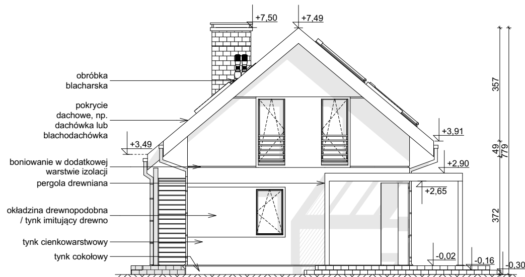
ELEWACJA BOCZNA
