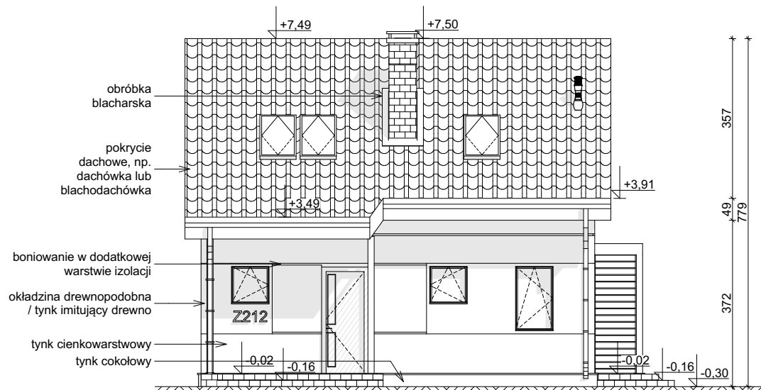
ELEWACJA FRONTOWA
