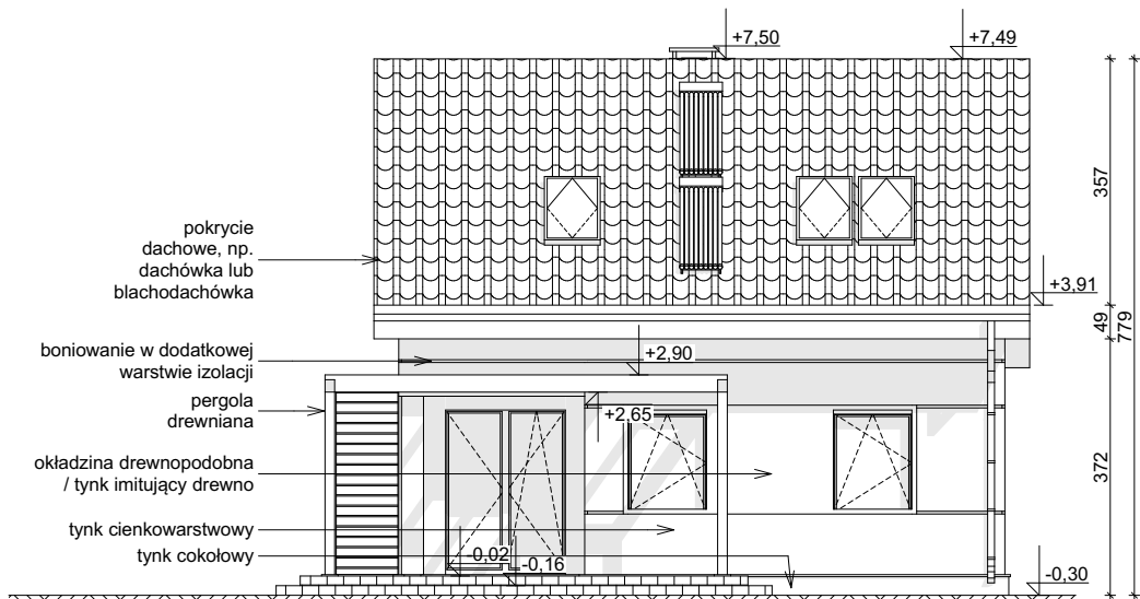
ELEWACJA OGRODOWA
