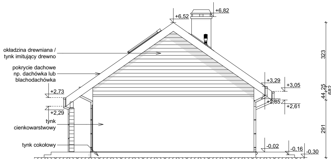
ELEWACJA BOCZNA
