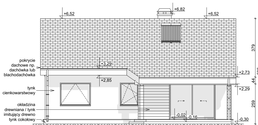
ELEWACJA OGRODOWA
