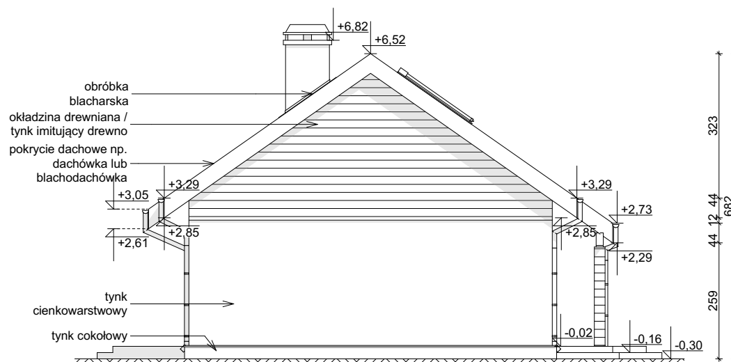
ELEWACJA BOCZNA
