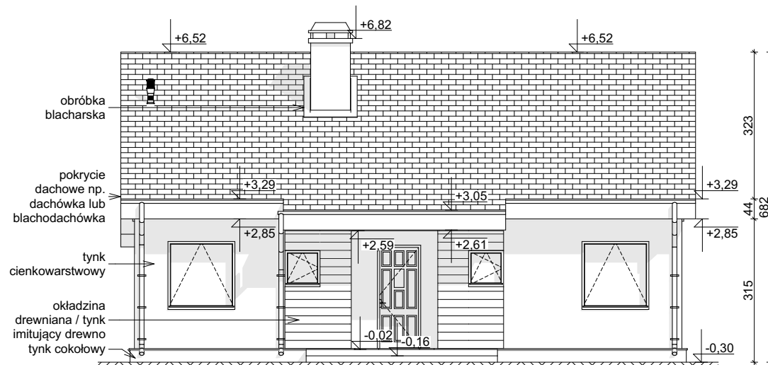
ELEWACJA FRONTOWA
