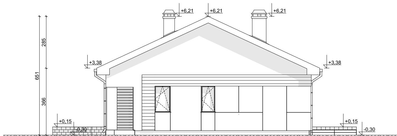
ELEVACJA BOCZNA
