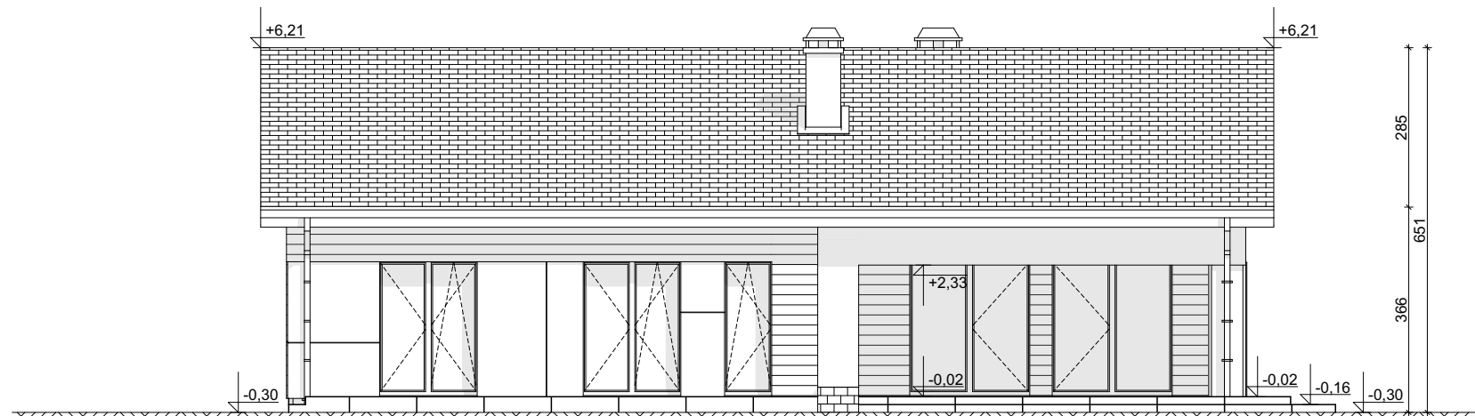
ELEVACJA OGRODOWA
